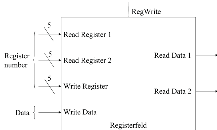
Abbildung 17.6: Zustandselement Registerfeld
