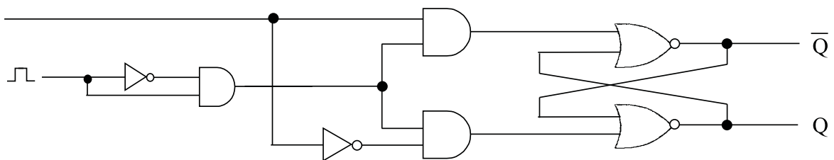
Abbildung 9.10: Pegelstände
