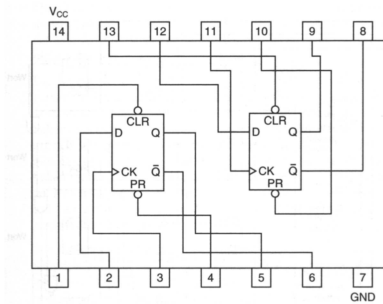
Abbildung 9.14: 2-Bit-Flip-Flop
