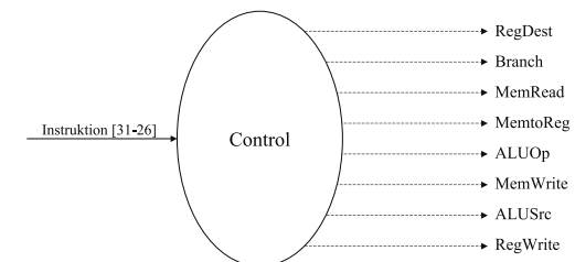
Abbildung 13.16: Control Element
