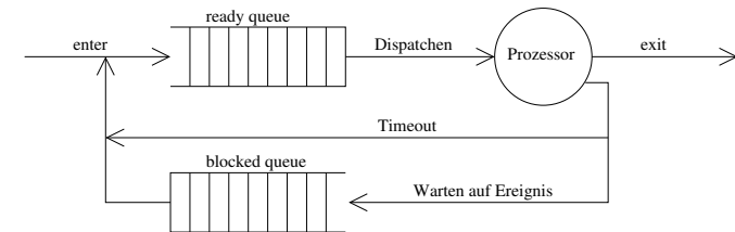
Abbildung 3.10: Warteschlangenmodell des 5-Zustands-Prozessmodells
