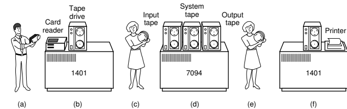
Abbildung 1.2: Erste Stapelverarbeitungssysteme
