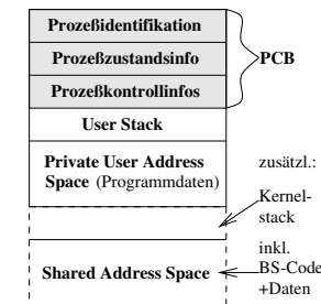
Abbildung 3.27: Prozeß-Image bei Integration der BS-Funktionen
