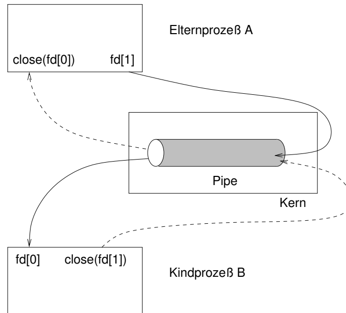
Abbildung 10.7: Daten fließen zum Kindprozeß
