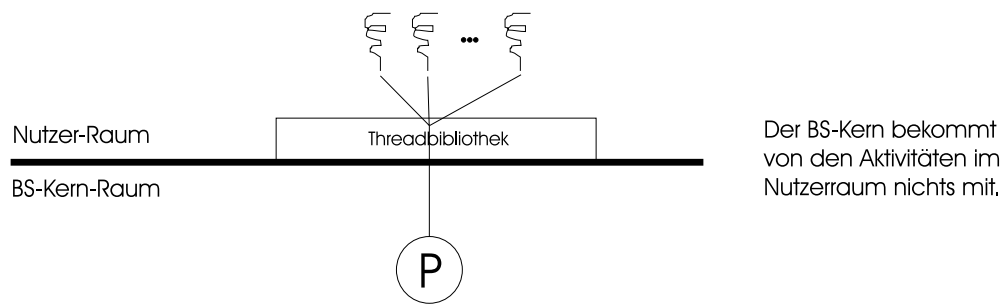
Abbildung 4.5: User-level-Thread-Modell 2
