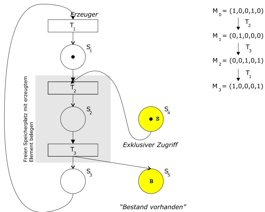
Abbildung 6.26: Entstehen eines Deadlocks
