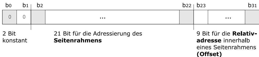
Abbildung 8.9: MI-Maschinenadresse
