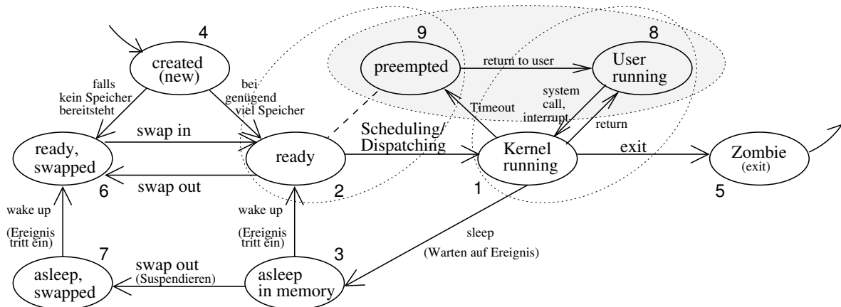
Abbildung 3.29: 9-Zustands-Modell (UNIX)
