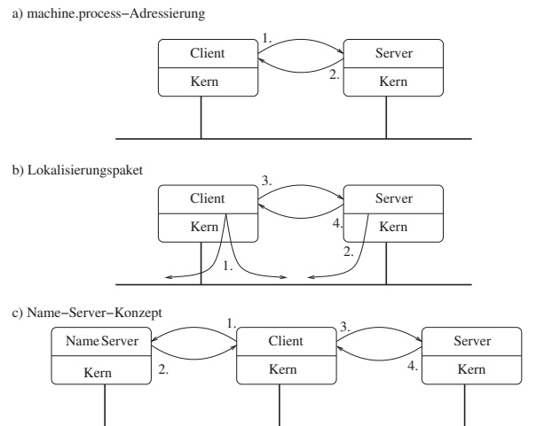
Abbildung 11.10: Varianten der Adressfindung
