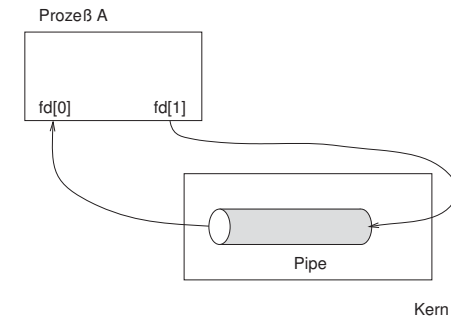
Abbildung 10.5: Einrichtung einer Pipe im Kernel
