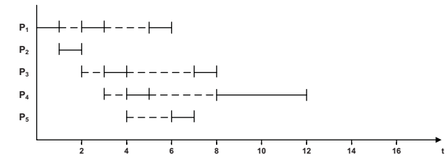
Abbildung 5.9: Beispiel mittlere Verweildauer für RR
