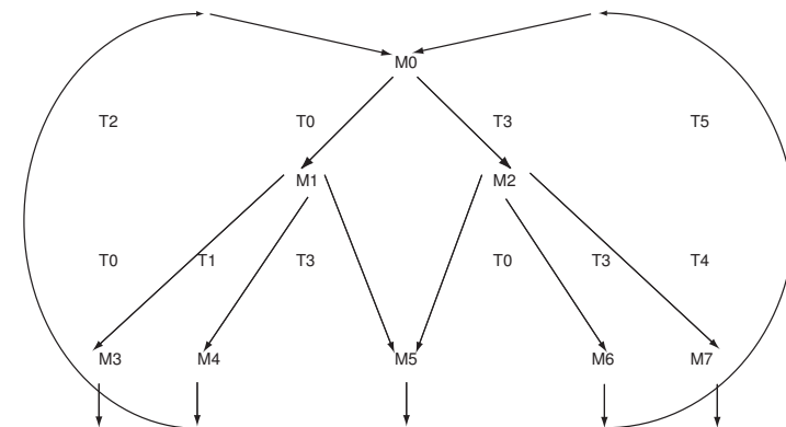
Abbildung 6.22: Vereinfachter Erreichbarkeitsgraph zum R/W-Problem
