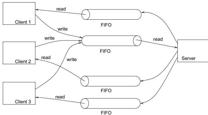
Abbildung 10.10: FIFO-Prinzip für drei Clients und einen Server
