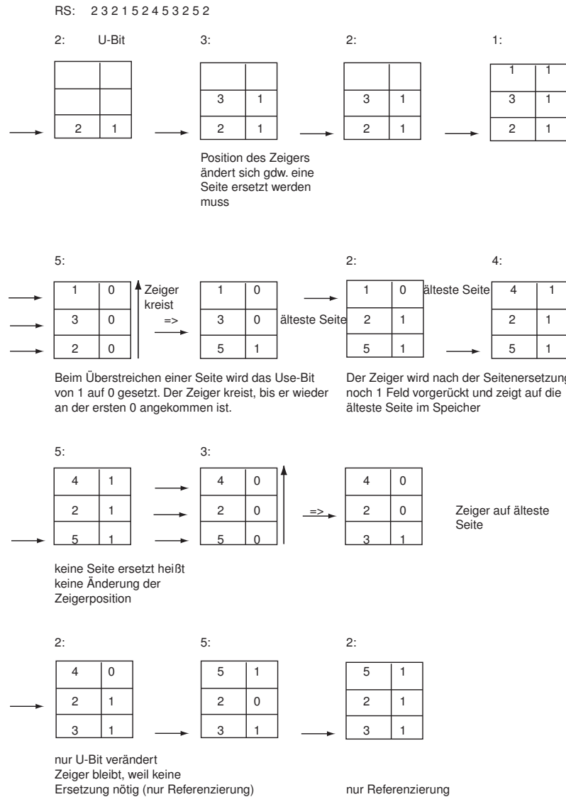
Abbildung 8.11: Beispiel zur Clock-Strategie
