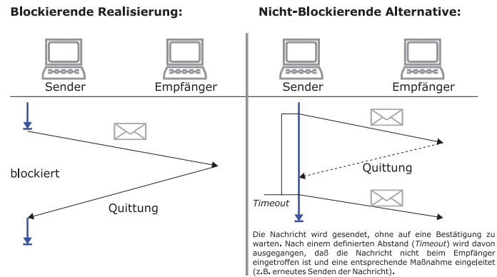
Abbildung 3.20: Blockierende und nicht-blockierende Realisierung von Signalen
