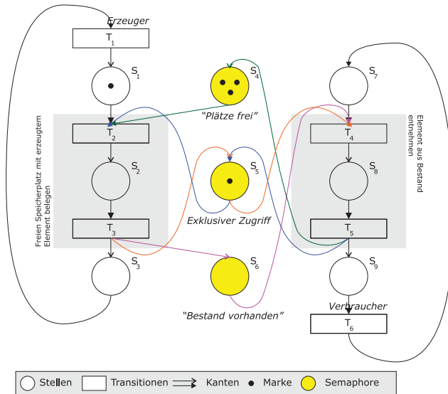
Abbildung 6.17: Petri-Netz zur Modellierung des Erzeuger/Verbraucher-Problems
