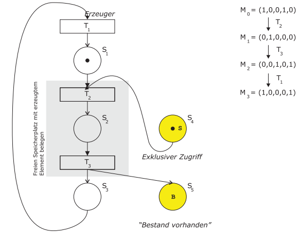
Abbildung 6.26: Entstehen eines Deadlocks
