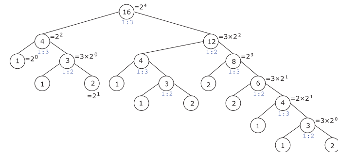
Abbildung 8.7: Veranschaulichung des Prinzips gewichteter Buddy Systeme
