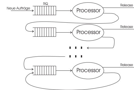
Abbildung 5.10: Implementierung und Abarbeitung eines Auftrags
