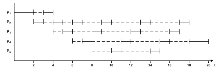
Abbildung 5.7: Beispiel mittlere Verweildauer für RR
