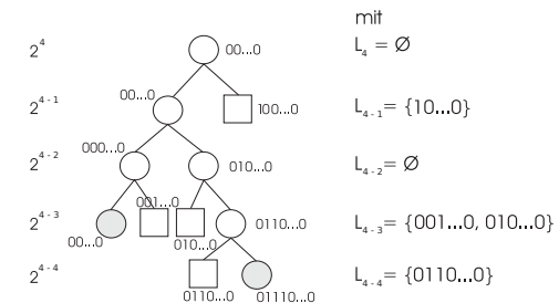
Abbildung 8.5: Adressierung in Buddy-Systemen
