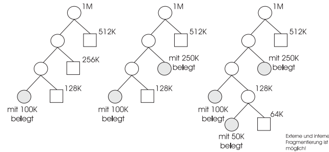
Abbildung 8.6: Fragmentierung bei Buddy-Systemen
