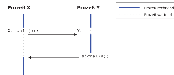
Abbildung 7.6: Ablaufsteuerung von zwei Prozessen mit Hilfe von Semaphoren
