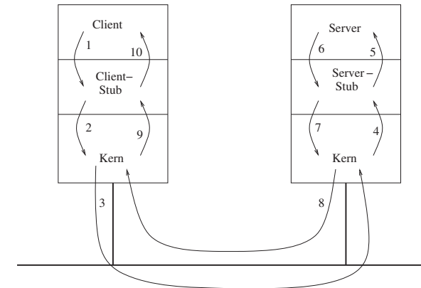
Abbildung 11.14: Ablauf eines RPCs
