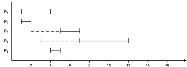
Abbildung 5.5: Beispiel mittlere Verweildauer für SRPT
