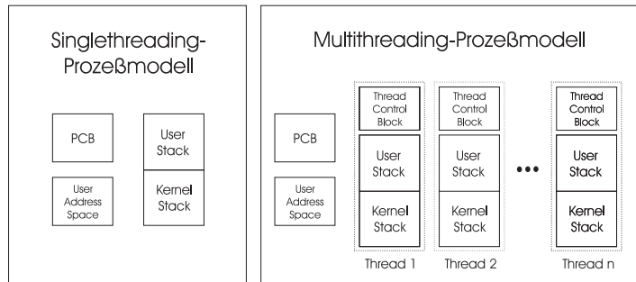
Abbildung 4.2: Singlethreading-Prozessmodell vs. Multithreading-Prozessmodell
