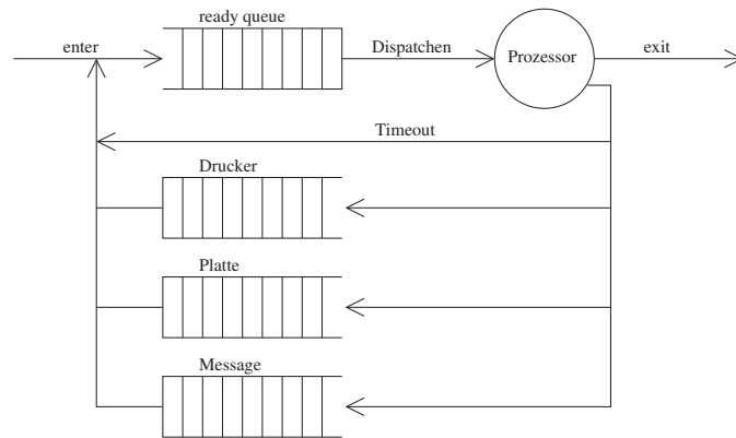
Abbildung 3.11: Implementierung mit mehreren Warteschlangen
