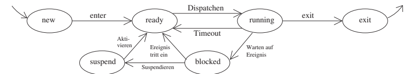
Abbildung 3.12: 5-Zustands-Modell mit Suspend
