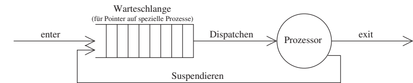
Abbildung 3.8: Warteschlangenmodell des 2-Zustand-Prozessmodells
