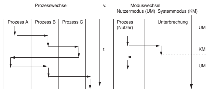
Abbildung 3.23: Prozess- und Moduswechsel
