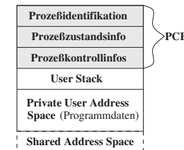
Abbildung 3.18: Struktur eines Prozesses im Hintergrundspeicher
