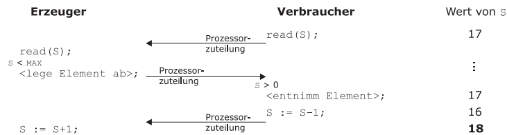
Abbildung 7.1: Ungeschützter Zugriff auf kritische Daten
