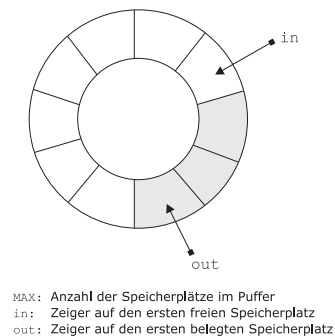
Abbildung 7.2: Darstellung eines einfachen Ringpuffers
