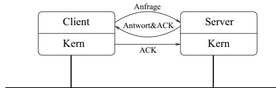
Abbildung 11.12: Bestätigung mittels piggy-backing
