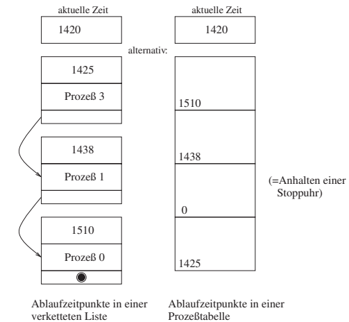
Abbildung 11.18: Verwaltung von Stoppuhren
