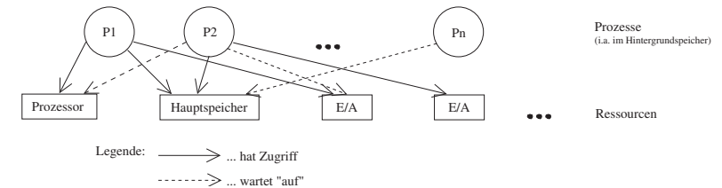
Abbildung 3.14: Verwaltung der Nutzung von Systemressourcen
