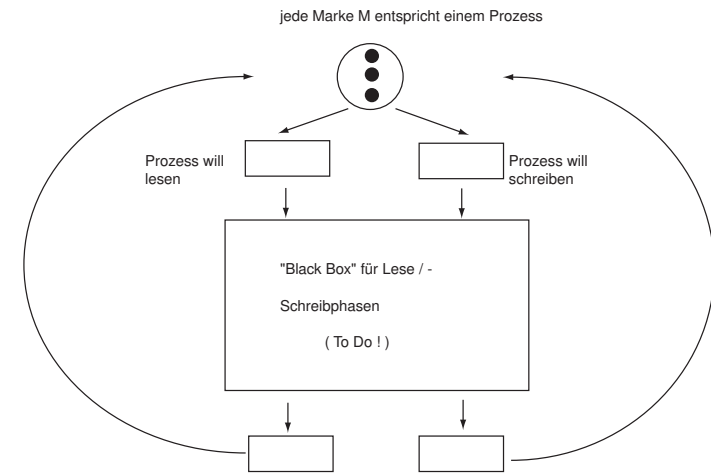
Abbildung 6.19: Einfaches Petri-Netz zum R/W-Problem
