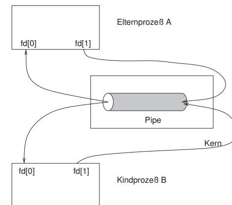
Abbildung 10.6: Grundsätzlicher Aufbau einer Pipekonstellation
