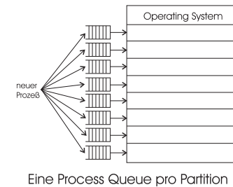
Abbildung 8.2: Technik der fixen Partitionierung
