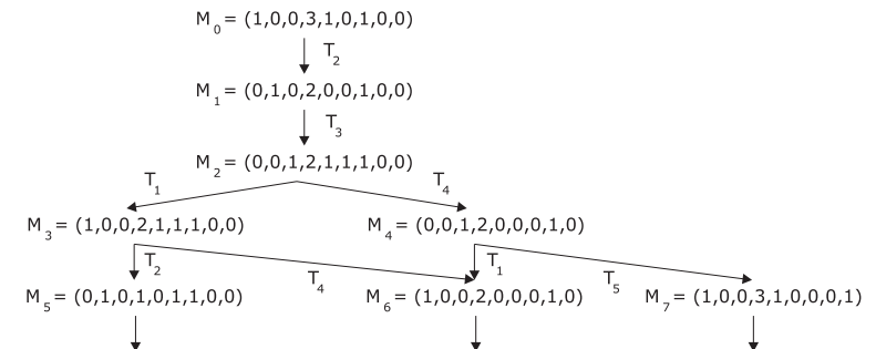
Abbildung 6.24: Erreichbarkeitsgraph zu Abbildung 6.17
