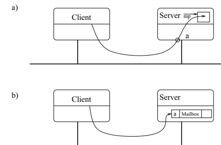
Abbildung 11.11: ungepufferte und gepufferte Primitive
