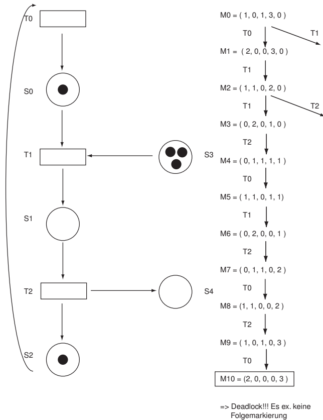
Abbildung 6.23: Beispiel eines Deadlocks
