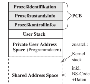
Abbildung 3.27: Prozeß-Image bei Integration der BS-Funktionen
