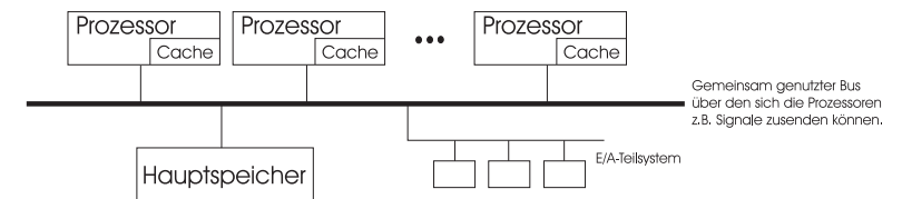
Abbildung 4.10: Prinzip der SMP-Organisation
