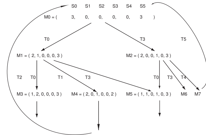
Abbildung 6.21: Erreichbarkeitsgraph zum R/W-Problem
