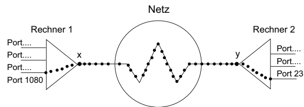
Abbildung 10.12: Das Socket Prinzip
