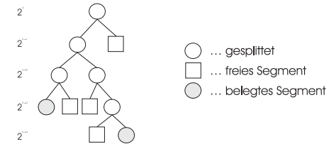
Abbildung 8.4: Beispiel für Buddy-Systeme
