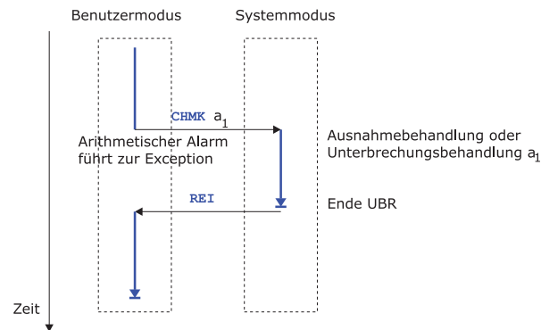
Abbildung 3.22: Prinzip einer Exception
