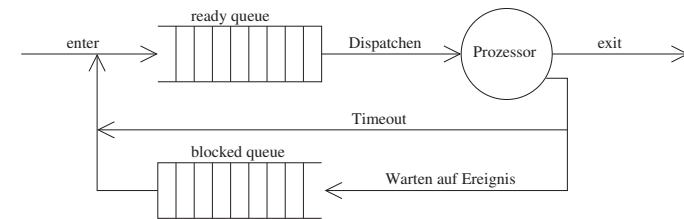
Abbildung 3.10: Warteschlangenmodell des 5-Zustand-Prozessmodells
