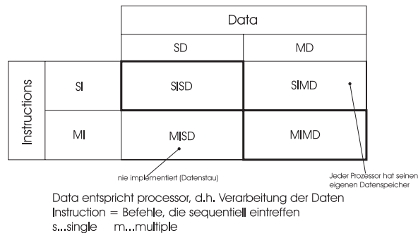
Abbildung 4.8: Einordnung von "Parallele Prozessoren"
