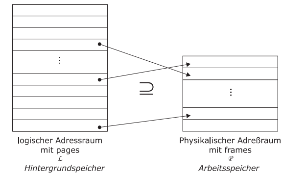
Abbildung 8.8: Abbildung zwischen frames und pages
