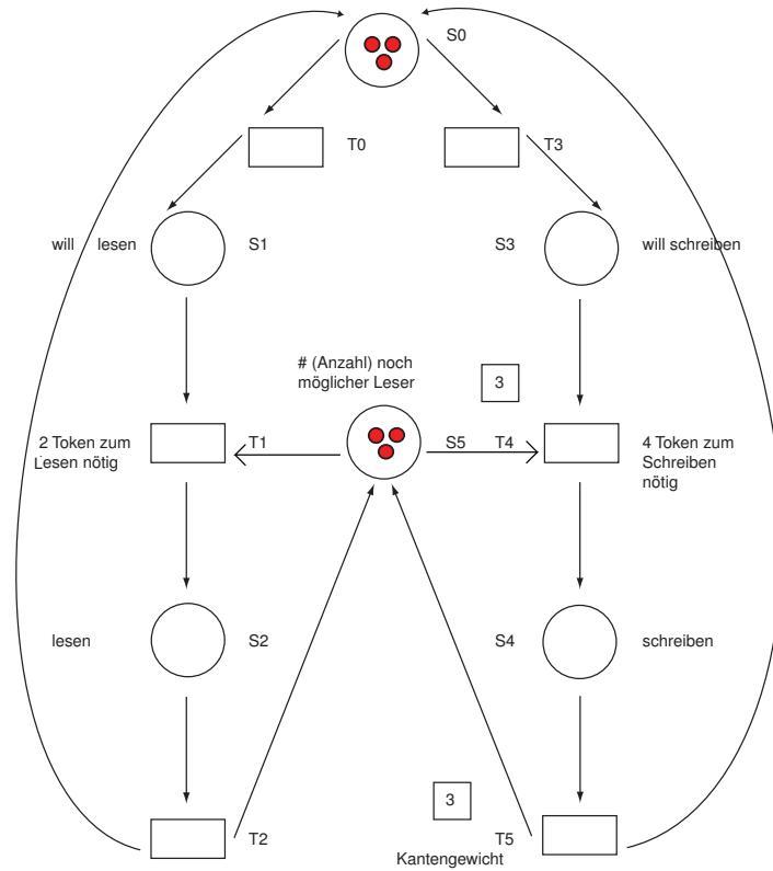
Abbildung 6.20: Fertiges Petri-Netz zum R/W-Problem
