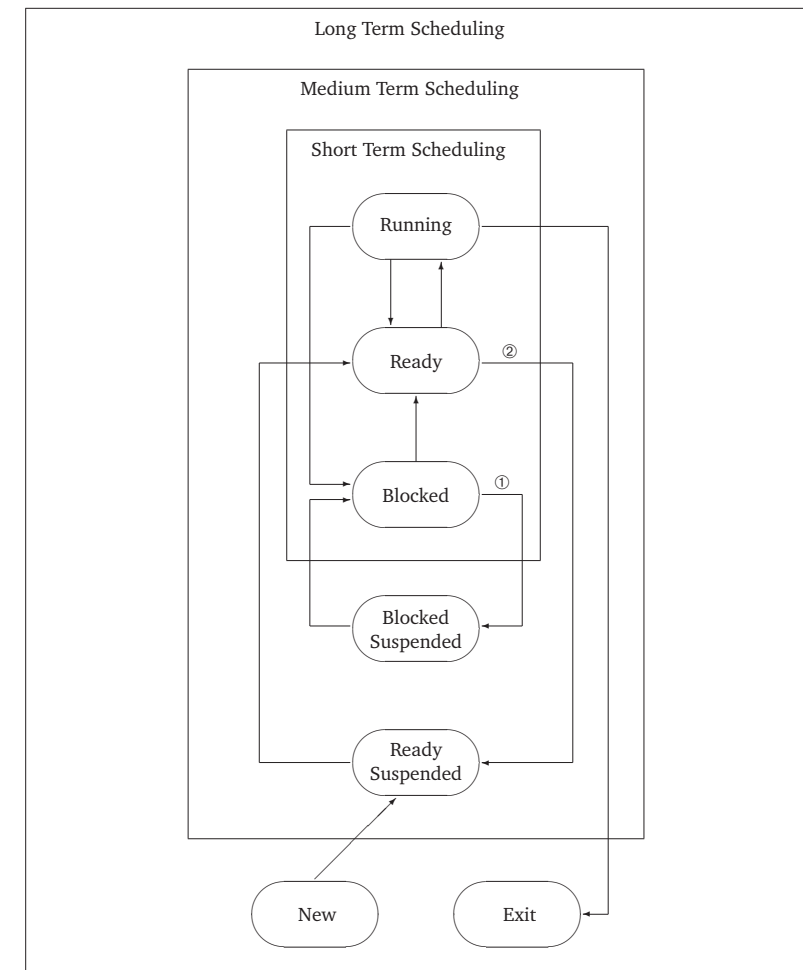
Abbildung 5.12: Visualisierung der hierarchischen Unterteilung der Scheduling-Arten
