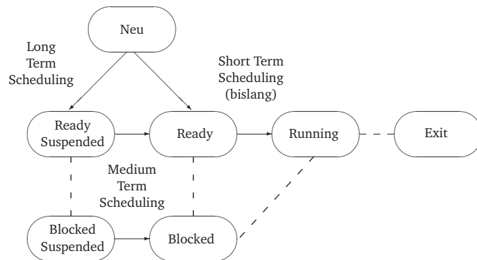
Abbildung 5.11: Zuordnung der Prozesszustände zu den Arten des Scheduling
