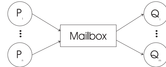
Abbildung 7.12: Indirekte Adressierung n:m
