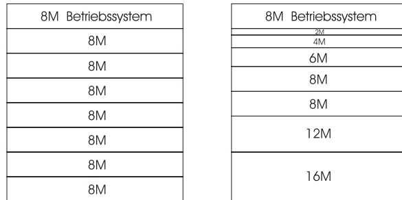
Abbildung 8.1: Beispiel für feste Partitionierung
