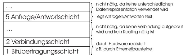
Abbildung 11.5: Der Protokollstapel des Client/Server-Modells
