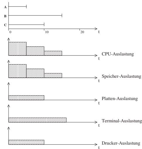
Abbildung 3.3: Ressourcennutzung bei verzahnter Ausführung von Jobs
