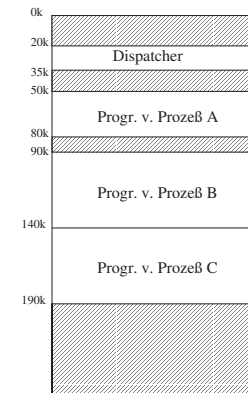
Abbildung 3.6: Speicherbelegung der drei Beispielprozesse
