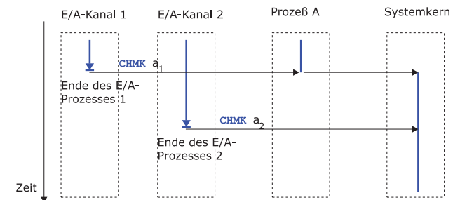
Abbildung 3.24: Beispiel für einen Unterbrechungskonflikt
