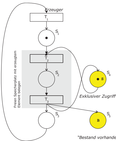
Abbildung 6.25: Entstehen eines Partial Deadlocks
