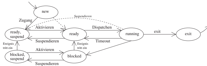
Abbildung 3.13: 7-Zustands-Prozessmodell
