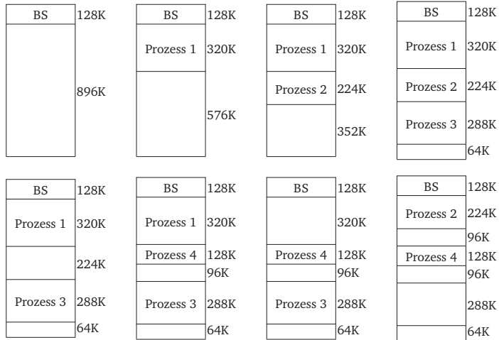
Abbildung 8.3: Dynamische Partitionierung
