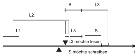
Abbildung 6.18: R/W-Problem
