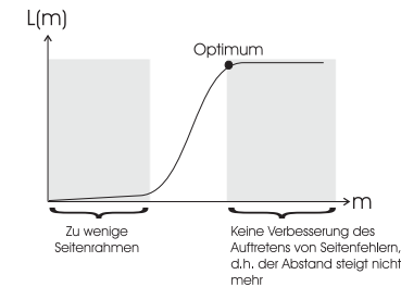
Abbildung 8.12: Lifetime-Funktion L(m)
