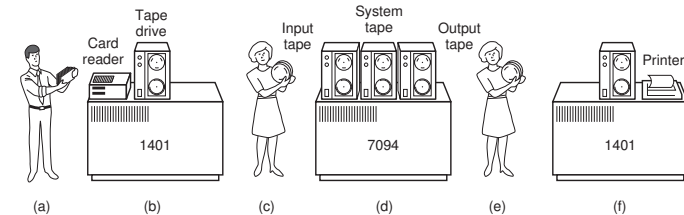
Abbildung 1.2: Erste Stapelverarbeitungssysteme
