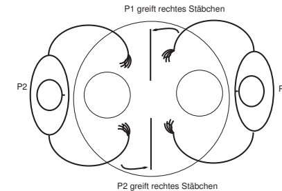
Abbildung 6.2: Beispiel Philosophenproblem
