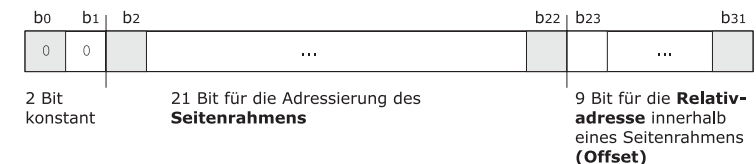
Abbildung 8.9: MI-Maschinenadresse
