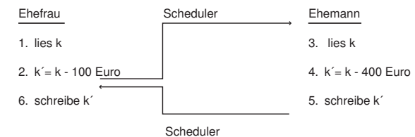
Abbildung 5.4: Programmbefehle
