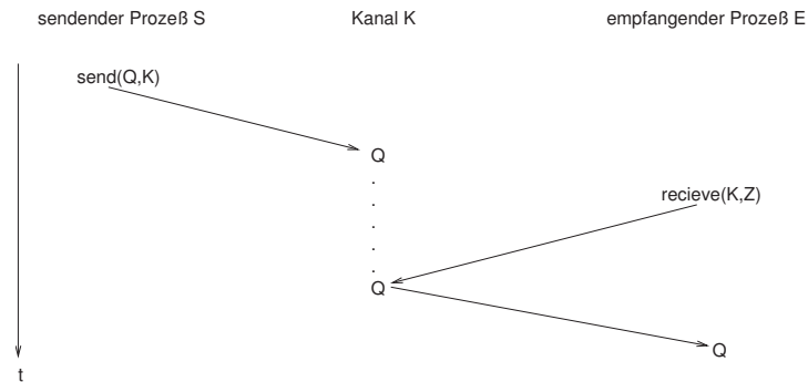
Abbildung 10.2: Send-Receive-Kommunikation (asynchron)
