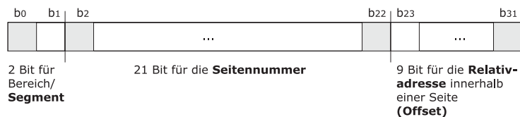
Abbildung 8.10: MI-Programmadresse
