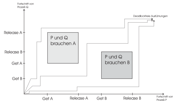
Abbildung 6.5: Prozeßfortschrittsdiagramm 2
