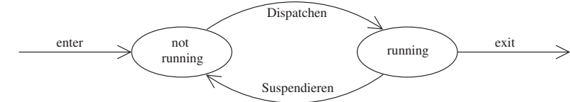
Abbildung 3.7: 2-Zustands-Prozessmodell
