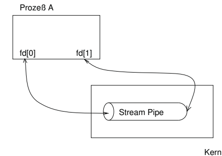
Abbildung 10.11: Stream-Pipe
