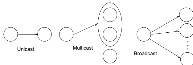
Abbildung 10.1: Grundlegende Verbindungstypen
