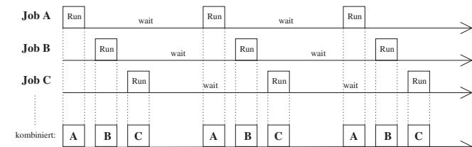
Abbildung 3.2: Pseudo-parallele Ausführung
