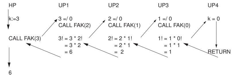
Abbildung 2.1: Sprünge bei rekursiven Unterprogrammaufrufen
