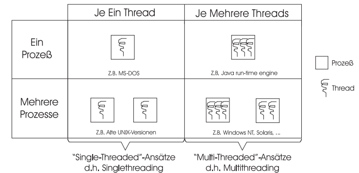
Abbildung 4.1: Die 4 Fälle beim Zusammenspiel von Threads und Prozessen
