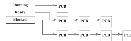
Abbildung 3.19: Implementierung des 5-Zustands-Prozessmodells
