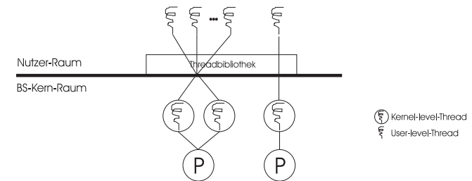
Abbildung 4.7: Thread-Modell für kombinierte Konzepte
