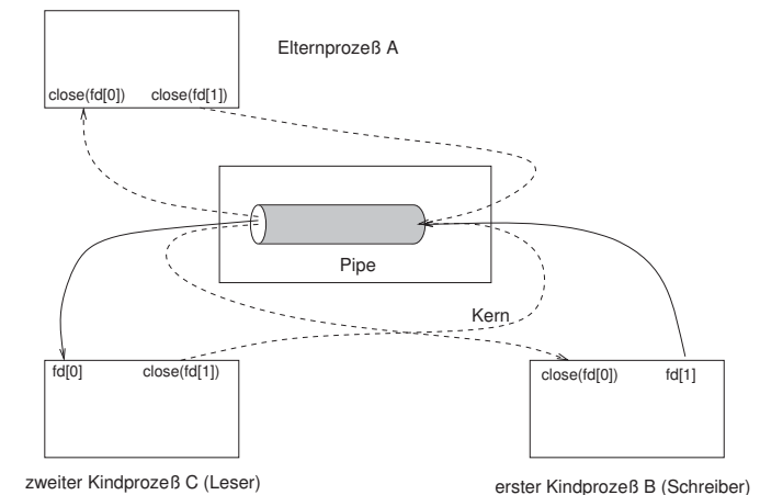
Abbildung 10.9: Kommunikation mit zwei Kindprozessen
