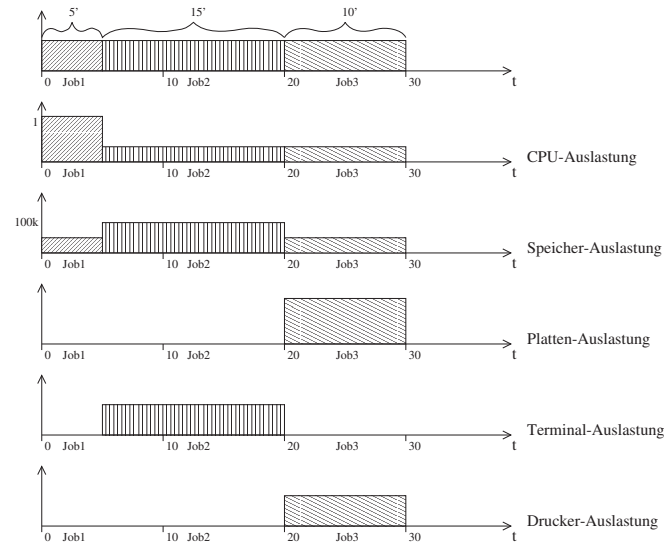
Abbildung 3.1: Ressourcennutzung bei sequenzieller Ausführung von Jobs
