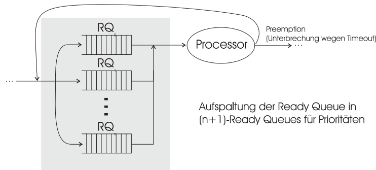
Abbildung 5.1: Aufspaltung in mehrere Ready-Queues für Prioritäten
