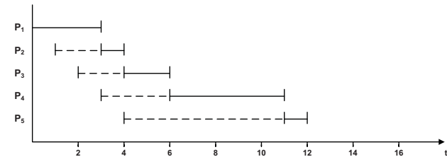
Abbildung 5.2: Beispiel mittlere Verweildauer für FCFS
