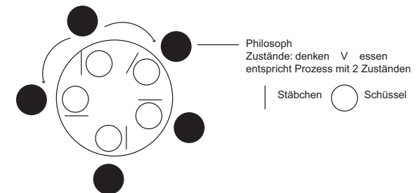
Abbildung 6.12: Philosophenproblem mit 5 Philosophen
