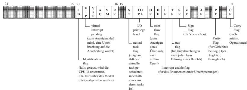
Abbildung 3.17: Struktur des Pentium-EFLAGS-Registers
