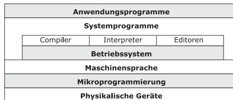
Abbildung 1.1: Logische Hierarchie in einem Rechner
