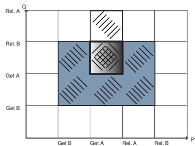
Abbildung 6.6: Bsp. Zustand ohne Deadlock
