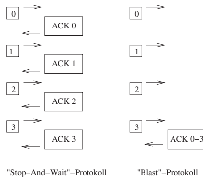
Abbildung 11.16: Möglichkeiten zur Bestätigung
