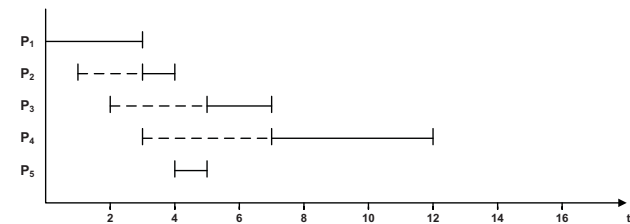
Abbildung 5.3: Beispiel mittlere Verweildauer für SJF
