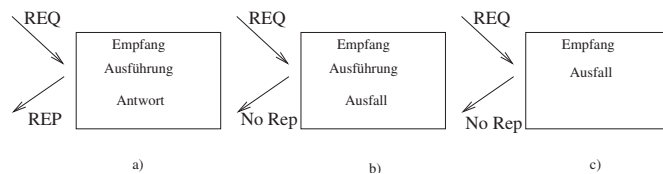
Abbildung 11.15: Serverausfall nach Erhalt einer Anfrage
