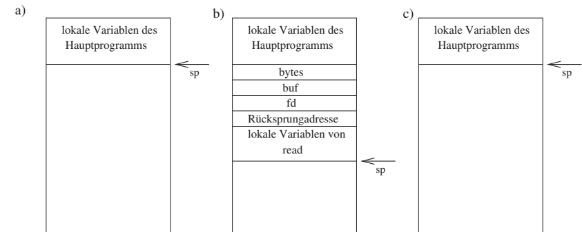
Abbildung 11.13: Stack bei lokalem Prozeduraufruf
