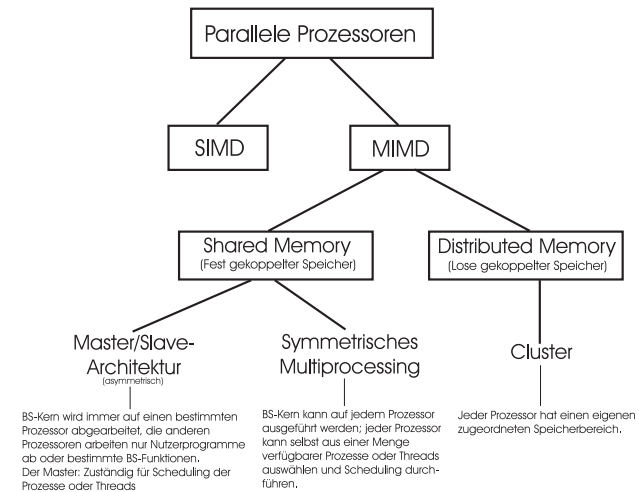
Abbildung 4.9: Parallele Prozessoren
