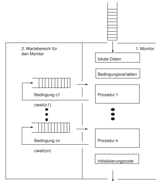
Abbildung 7.8: Monitor
