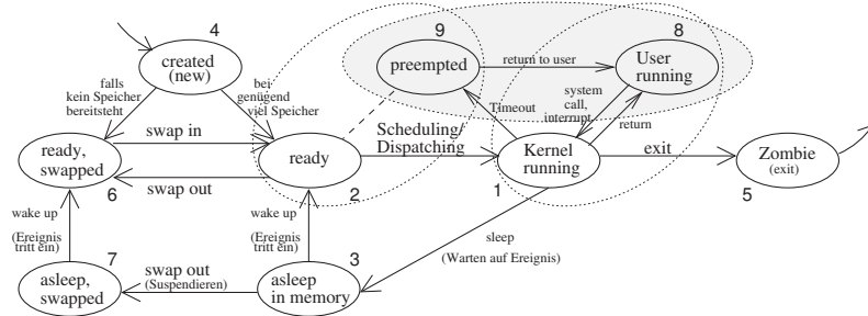
Abbildung 3.29: 9-Zustands-Modell (UNIX)
