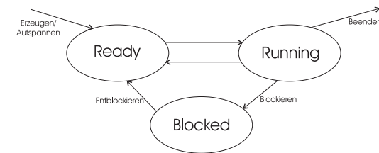
Abbildung 4.3: Thread-Zustandsübergangsdiagramm
