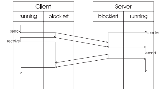
Abbildung 11.9: Blockierende Kommunikationsprimitive
