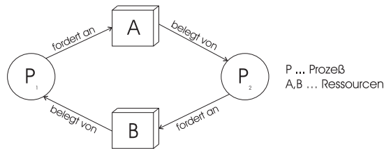
Abbildung 6.7: Circular Wait
