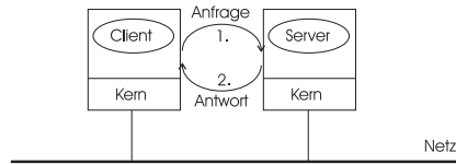
Abbildung 11.4: Das Client/Server-Modell
