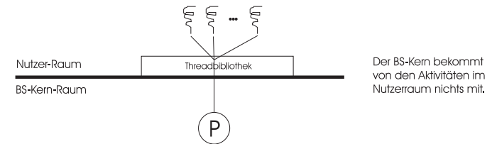
Abbildung 4.5: User-level-Thread-Modell 2
