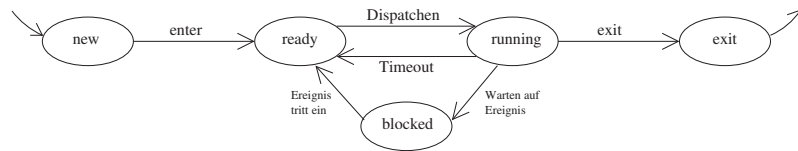
Abbildung 3.9: 5-Zustands-Prozessmodell
