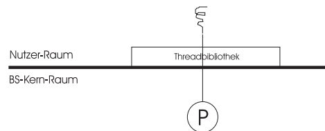
Abbildung 4.4: User-level-Thread-Modell
