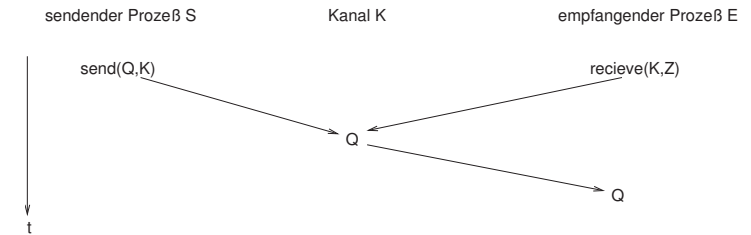
Abbildung 10.4: Synchrone Kommunikation
