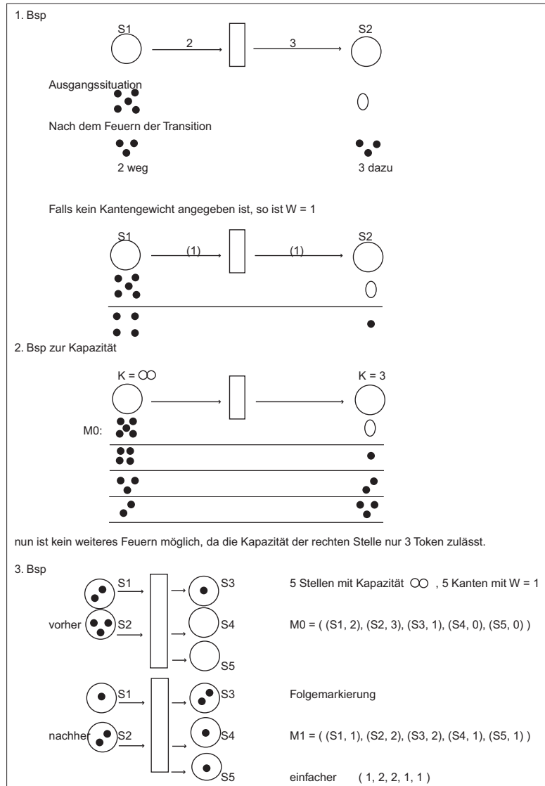
Abbildung 6.11: Stellen-Transitionssysteme
