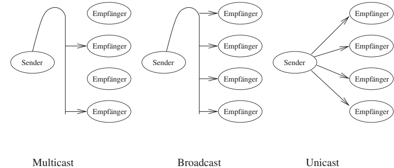
Abbildung 11.20: Verschiedene Übertragungsverfahren
