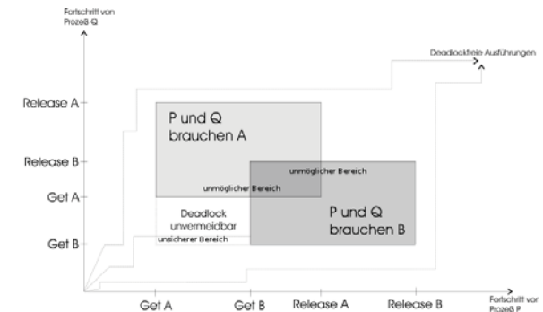
Abbildung 6.4: Prozeßfortschrittsdiagramm 1
