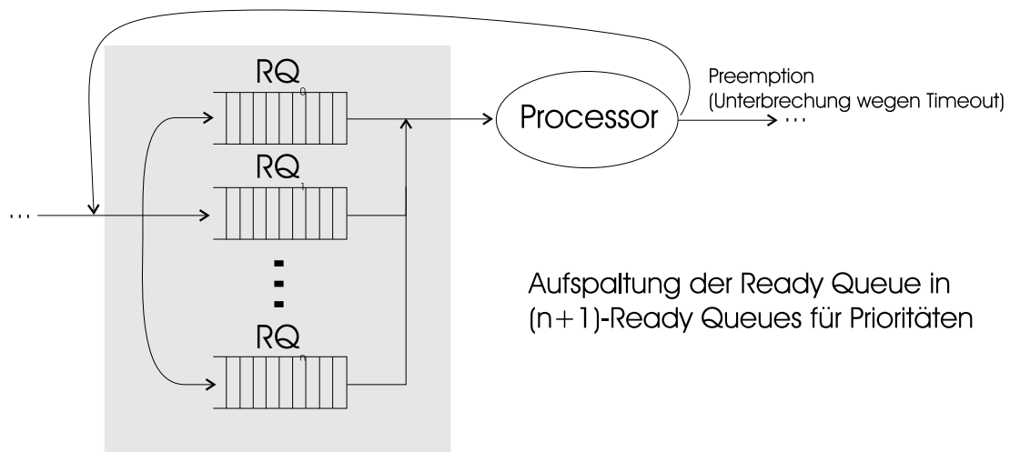
Abbildung 5.1: Aufspaltung in mehrere Ready-Queues für Prioritäten
