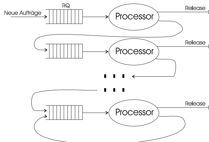
Abbildung 5.10: Implementierung und Abarbeitung eines Auftrags
