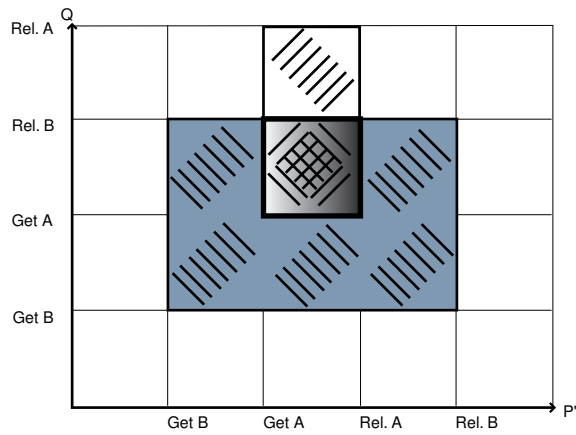
Abbildung 6.6: Bsp. Zustand ohne Deadlock
