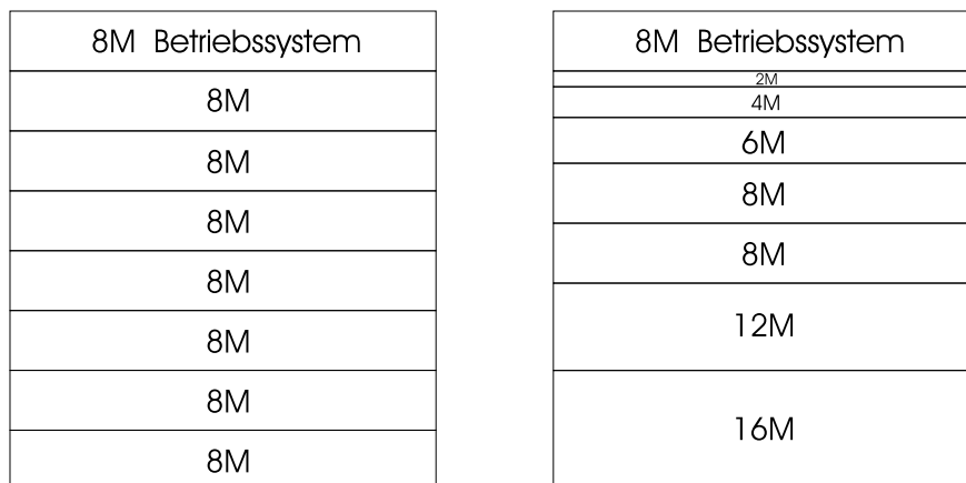
Abbildung 8.1: Beispiel für feste Partitionierung
