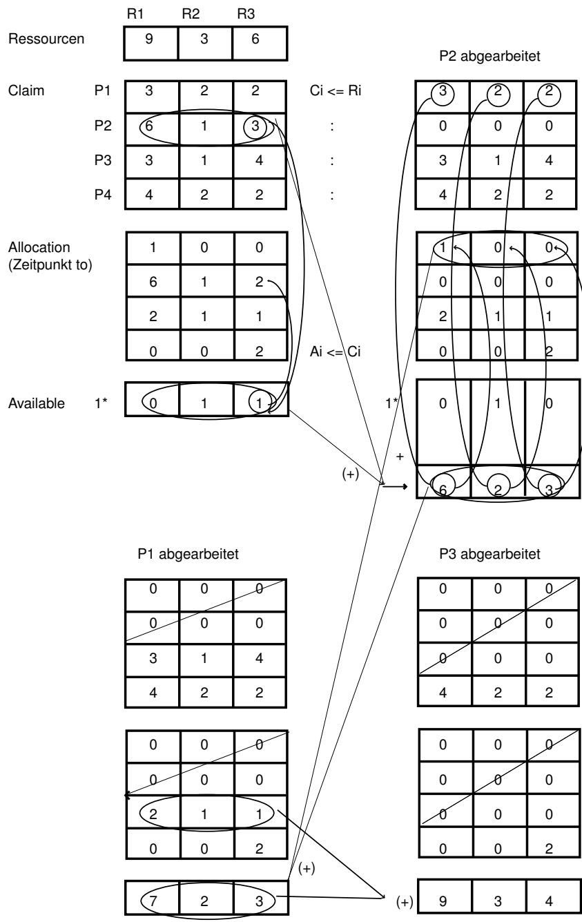
Abbildung 6.8: Beispiel eines sicheren Zustandes
