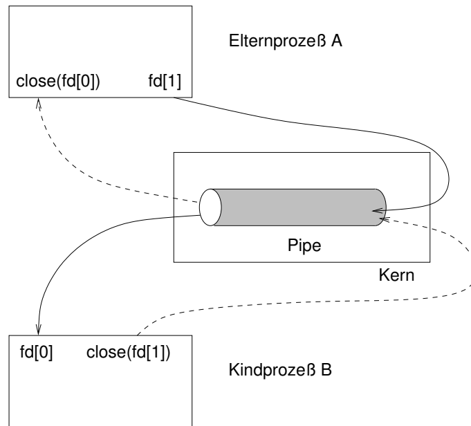
Abbildung 10.7: Daten fließen zum Kindprozess
