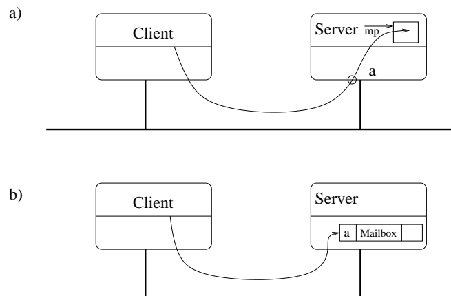
Abbildung 11.11: ungepufferte und gepufferte Primitive
