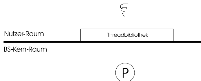
Abbildung 4.4: User-level-Thread-Modell
