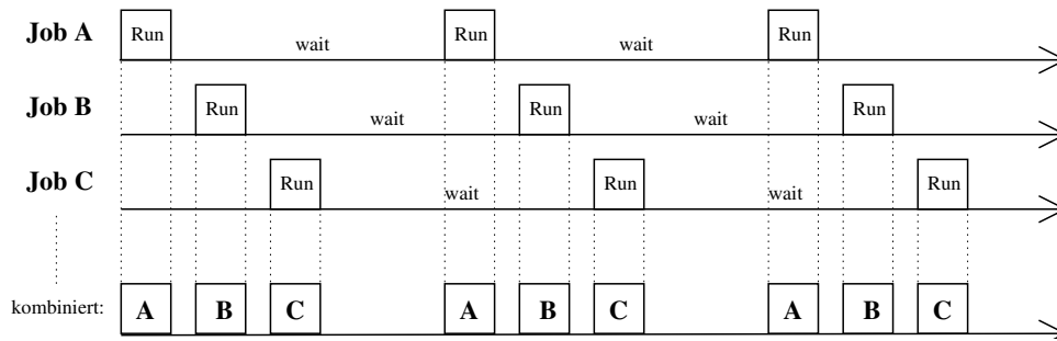
Abbildung 3.2: Pseudo-parallele Ausführung
