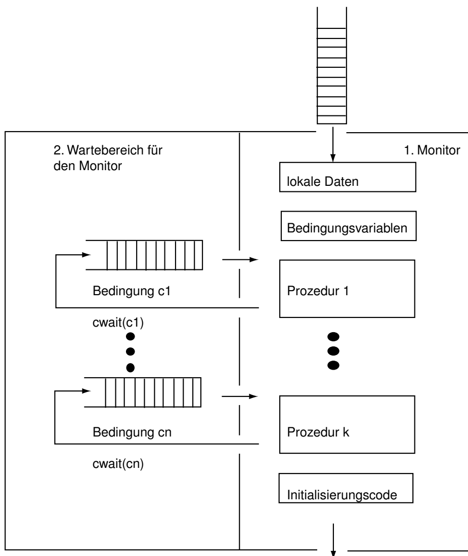
Abbildung 7.8: Monitor
