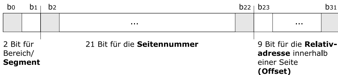
Abbildung 8.10: MI-Programmadresse
