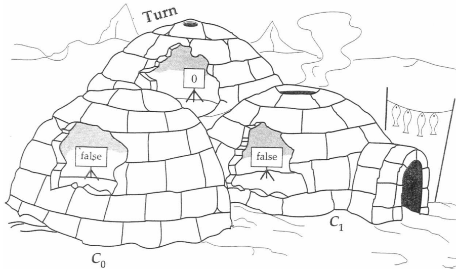
Abbildung 7.5: Die korrekte Lösung: Schiedsrichteriglo mit Variable turn zeigt an, welcher Prozess Vorrang hat.
