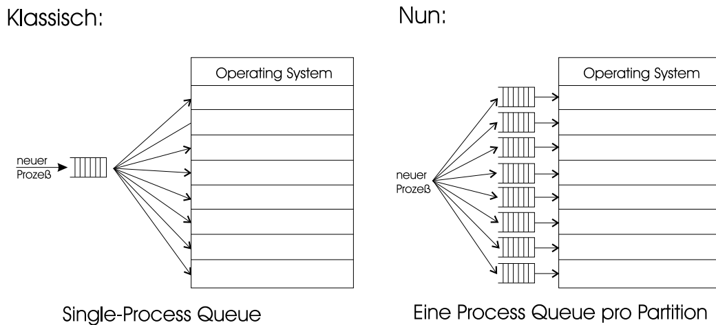
Abbildung 8.2: Technik der fixen Partitionierung
