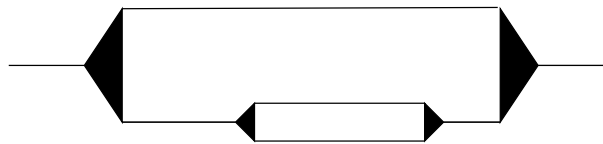
Abbildung 3.4: FORK-Darstellung
