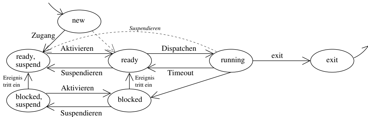
Abbildung 3.13: 7-Zustands-Prozessmodell
