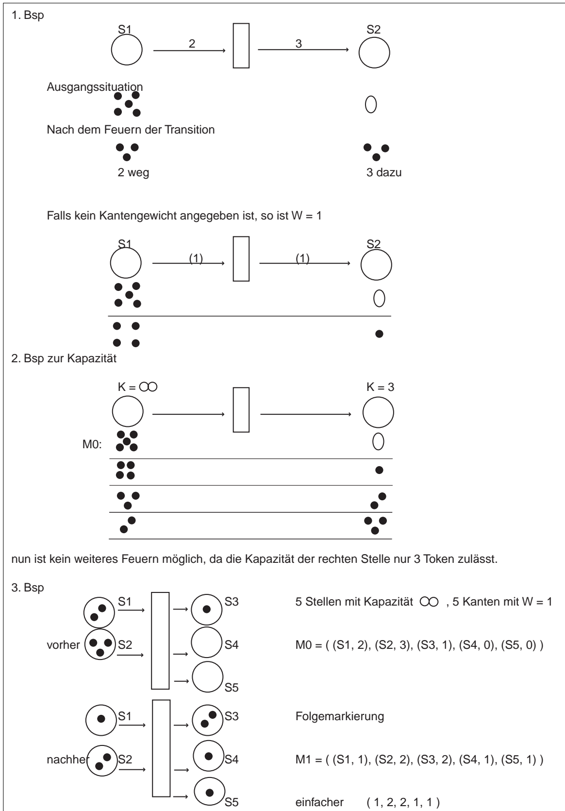
Abbildung 6.11: Stellen-Transitionssysteme
