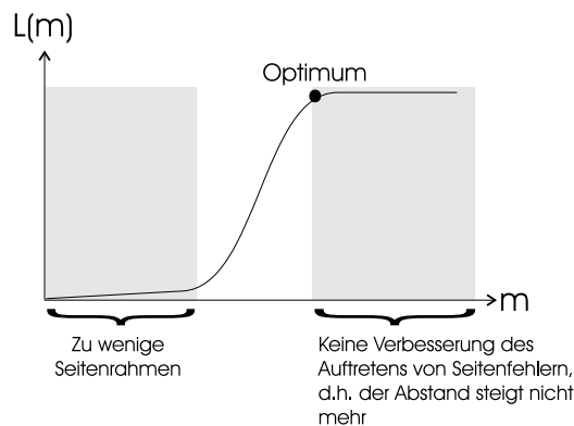
Abbildung 8.12: Lifetime-Funktion L(m)
