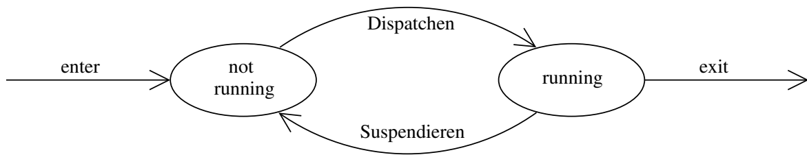
Abbildung 3.7: 2-Zustands-Prozessmodell
