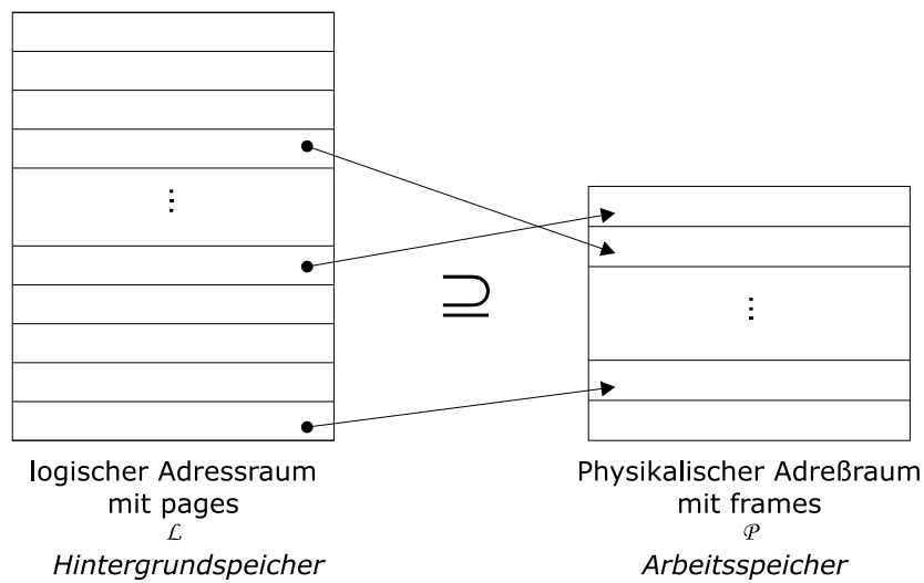
Abbildung 8.8: Abbildung zwischen frames und pages
