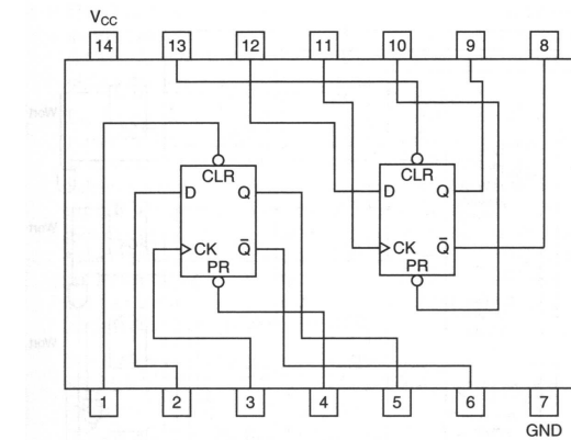
Abbildung 9.14: 2-Bit-Flip-Flop
