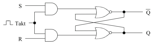
Abbildung 9.7: Getaktetes SR-Latch
