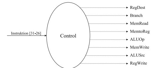
Abbildung 17.16: Control Element
