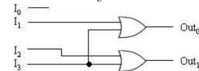
Abbildung 7.10: 4-to-2-Encoder
