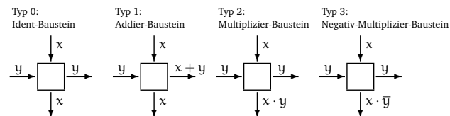
Abbildung 7.18: verschiedene Gitterpunkt-Typen
