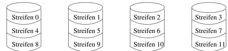
Abbildung 16.5: RAID-System für Level 0, das aus 4 Einzelplatten besteht
