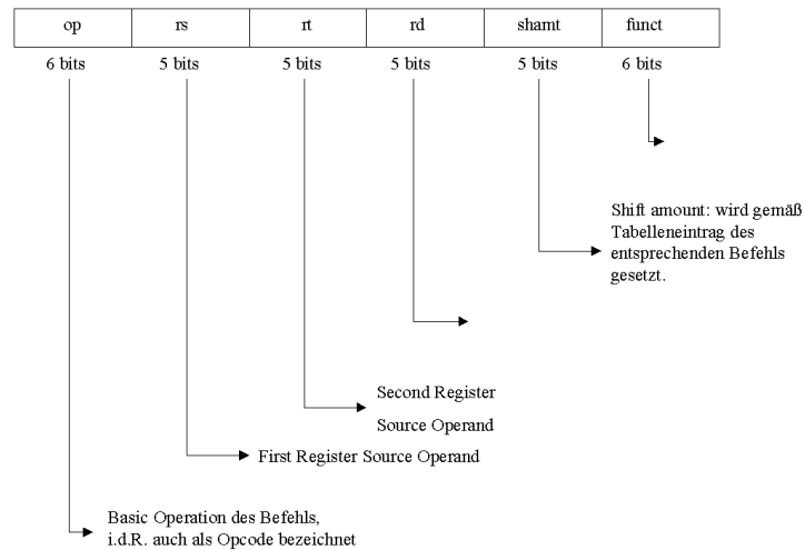
Abbildung 6.1: MIPS-Befehl
