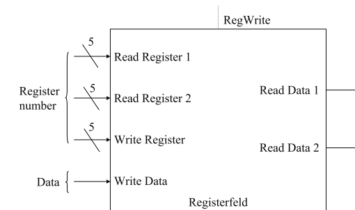
Abbildung 17.6: Zustandselement Registerfeld
