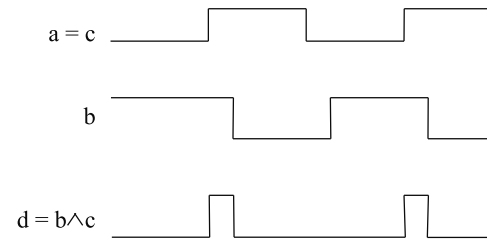
Abbildung 9.10: Pegelstände
