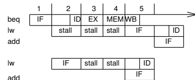
Abbildung 18.4: sequentielle Ausführung
