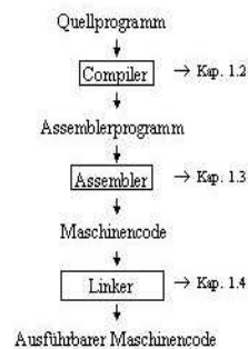
Abbildung 5.3: Compilierungsphasen
