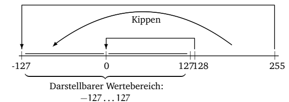
Abbildung 8.2: Vorzeichen/Betrag-Darstellung
