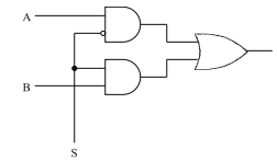
Abbildung 7.12: 2-Eingaben-Multiplexer
