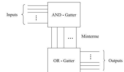
Abbildung 7.19: PLA
