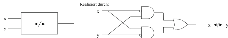
Abbildung 7.5: Antivalenz
