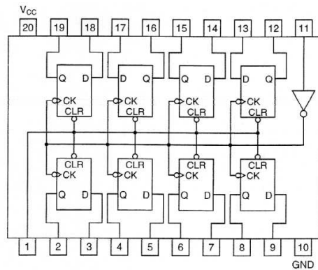
Abbildung 9.15: 8-Bit-Flip-Flop
