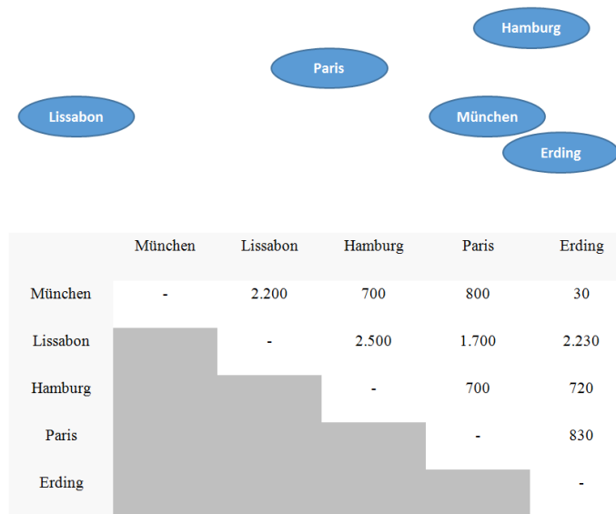
Abbildung 10.2: Das Traveling-Salesman-Problem für 5 Städte
