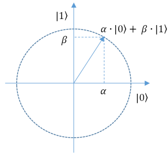
Abbildung 11.2: Die Superposition als Vektor.
