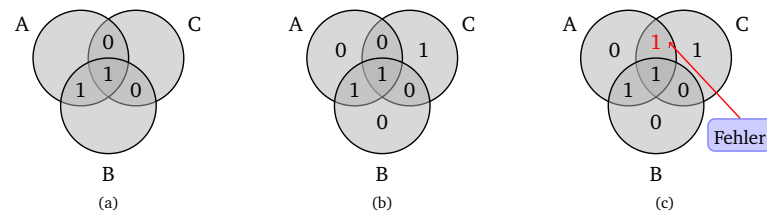
Abbildung 14.2: Venn-Diagramm
