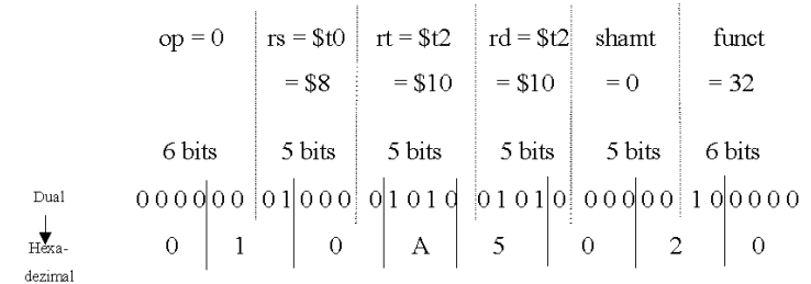
Abbildung 6.2: Codierung
