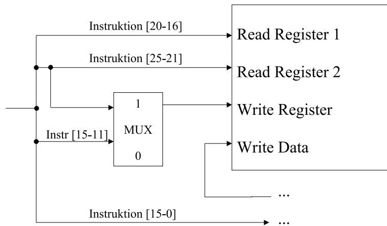
Abbildung 17.15: Einfügen des Multiplexers
