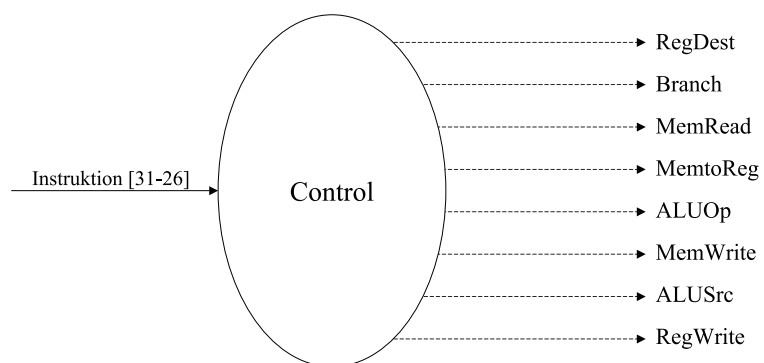
Abbildung 17.16: Control Element
