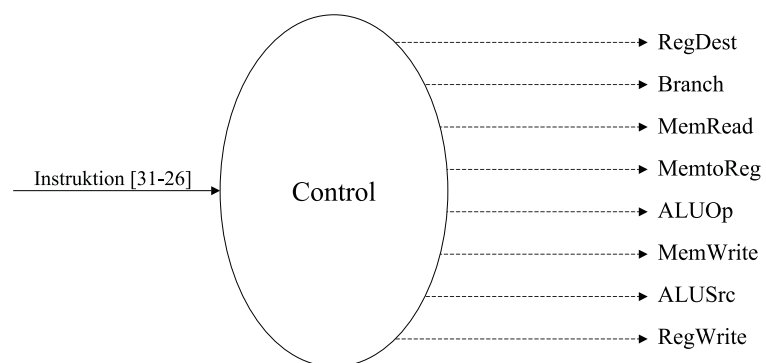
Abbildung 13.16: Control Element
