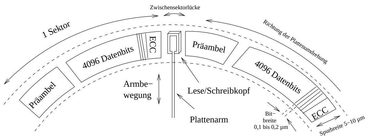
Abbildung 12.4: Zwei Sektoren auf einer Plattenspur
