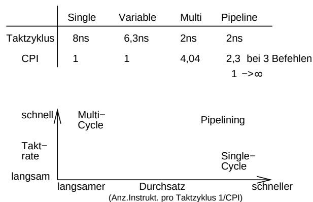
Abbildung 14.3: Vergleich: Taktrate / Durchsatz (CPI)
