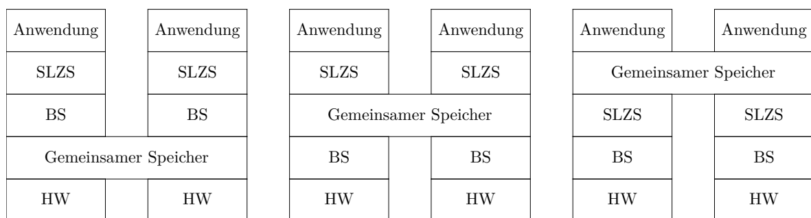
Abbildung 16.3: Hybrides System
