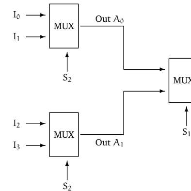
Abbildung 7.15: 4-Eingaben-Multiplexer durch 3 2-MUX realisiert
