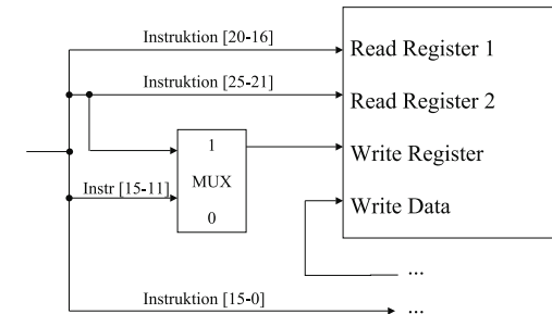
Abbildung 13.15: Einfügen des Multiplexers
