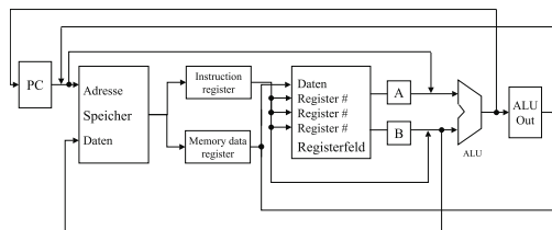
Abbildung 13.17: Grundprinzip der Multicycle Architektur
