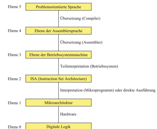
Abbildung 15.2: Die Struktur eines Computers mit 6 Ebenen
