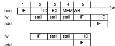
Abbildung 14.4: sequentielle Ausführung
