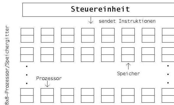
Abbildung 16.6: Arrayprozessor
