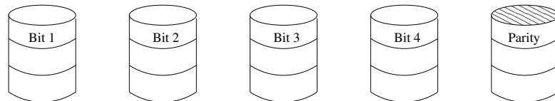
Abbildung 12.8: RAID-System für Level 3 mit einem Paritätsbit
