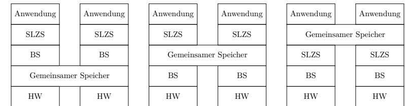
Abbildung 16.3: Hybrides System
