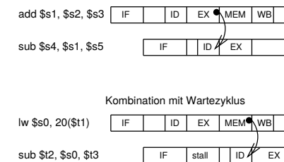
Abbildung 14.6: Auflösung des Datenhazard beim Pipelining
