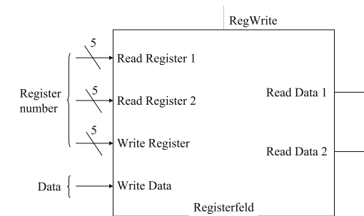
Abbildung 13.6: Zustandselement Registerfeld
