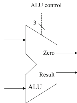
Abbildung 13.9: ALU
