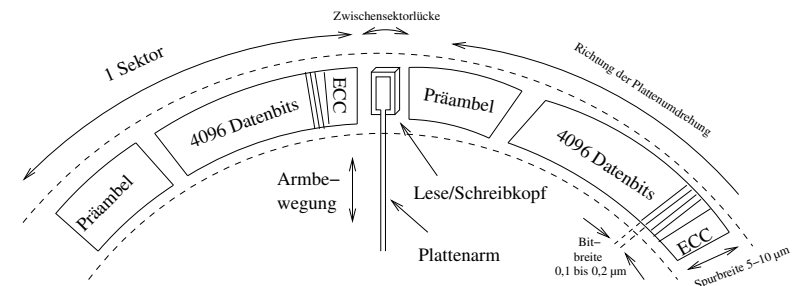
Abbildung 12.4: Zwei Sektoren auf einer Plattenspur
