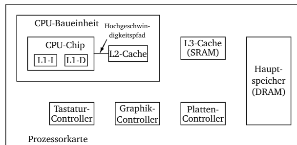
Abbildung 11.2: Prozessorkarte mit drei Cache-Ebenen
