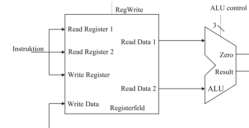
Abbildung 13.10: Datenpfad für R-Type
