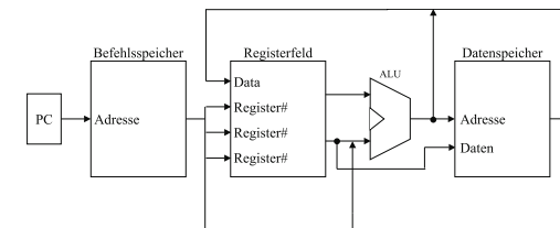
Abbildung 13.1: logische Funktionsweise des Prozessors
