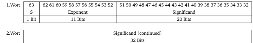
Abbildung 8.7: Bitaufteilung bei Double
