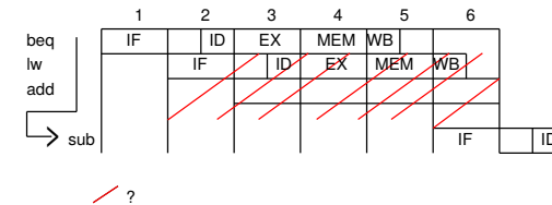
Abbildung 14.5: Verzweigungsvorhersage
