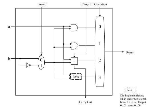
Abbildung 13.7: Aufbau der ALU beim MIPS
