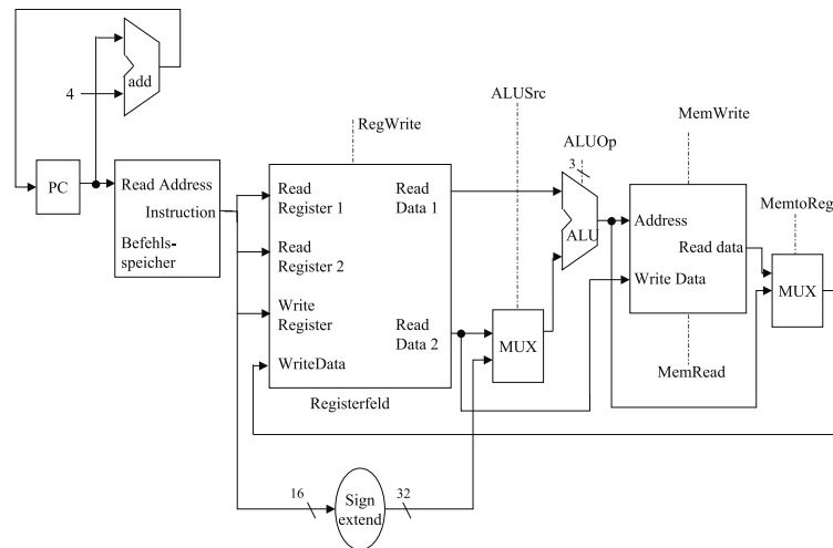
Abbildung 13.14: Datenpfad
