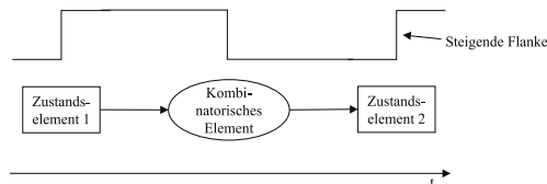
Abbildung 13.2: Zeitliche Abhängigkeit
