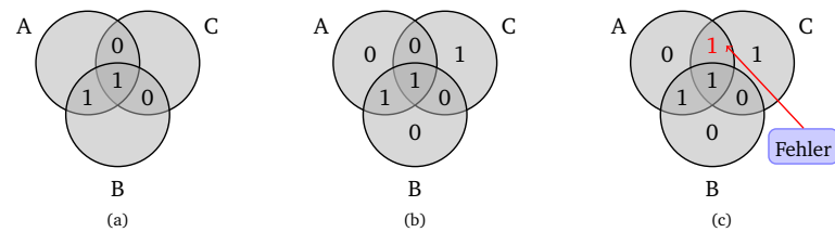
Abbildung 10.2: Venn-Diagramm
