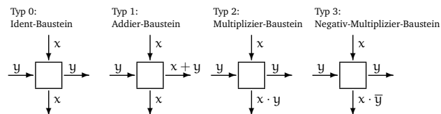
Abbildung 7.18: verschiedene Gitterpunkt-Typen
