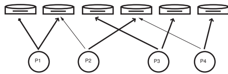
Abbildung 6.3: Beispiel mit 4 Prozessen. Dicke Pfeile deuten an, dass ein Prozess ein Betriebsmittel hält, dünne Pfeile, dass ein Prozess auf ein Betriebsmittel wartet.
