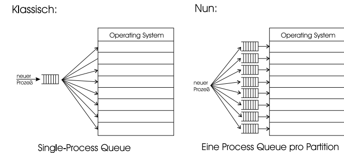
Abbildung 8.2: Technik der fixen Partitionierung
