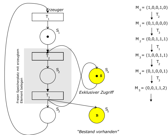
Abbildung 6.25: Entstehen eines Partial Deadlocks
