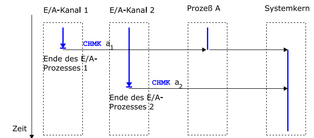
Abbildung 3.24: Beispiel für einen Unterbrechungskonflikt
