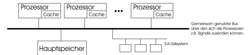
Abbildung 4.10: Prinzip der SMP-Organisation
