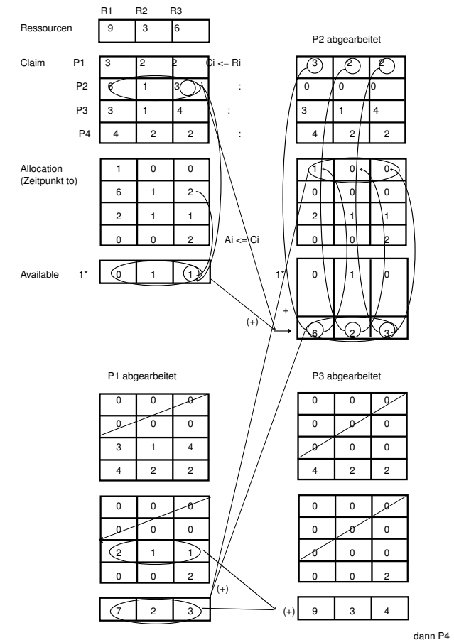
Abbildung 6.8: Beispiel eines sicheren Zustandes
