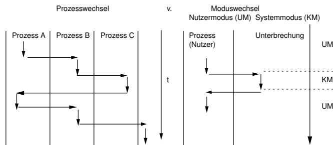
Abbildung 3.23: Prozess- und Moduswechsel
