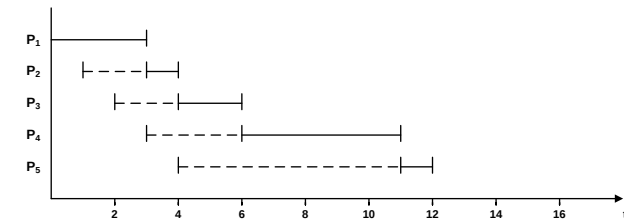
Abbildung 5.2: Beispiel mittlere Verweildauer für FCFS
