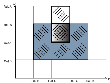
Abbildung 6.6: Bsp. Zustand ohne Deadlock
