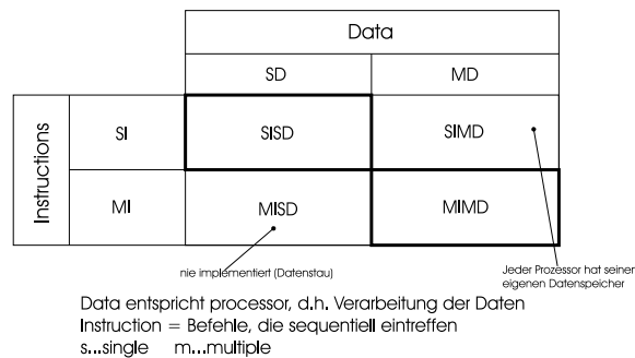
Abbildung 4.8: Einordnung von "Parallele Prozessoren"
