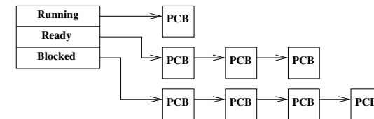
Abbildung 3.19: Implementierung des 5-Zustands-Prozessmodells
