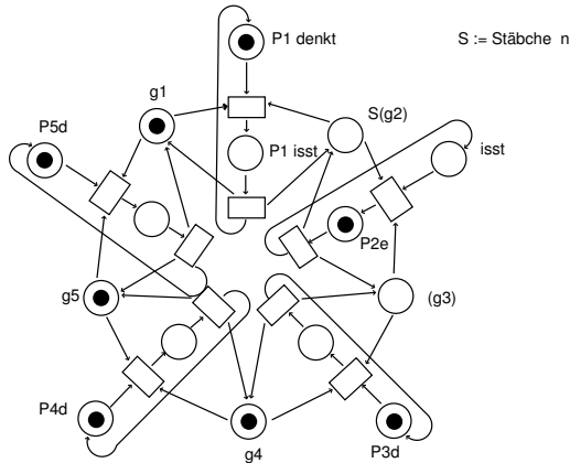
Abbildung 6.13: Petri-Netz zum Philosophenproblem mit 5 Philosophen
