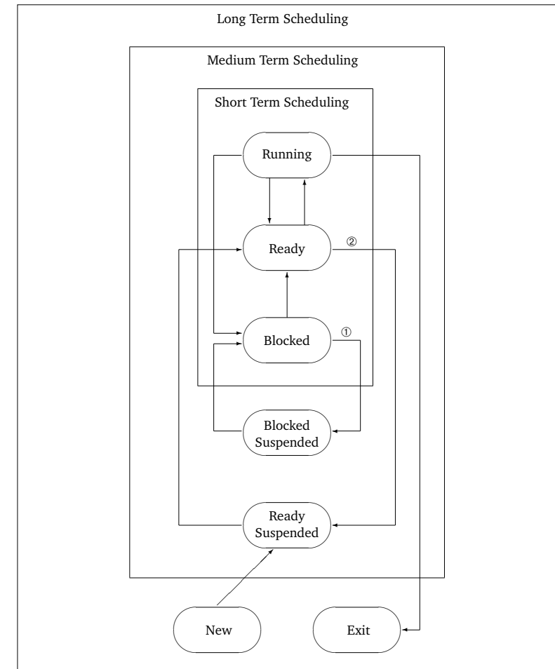
Abbildung 5.12: Visualisierung der hierarchischen Unterteilung der Scheduling-Arten
