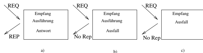
Abbildung 11.15: Serverausfall nach Erhalt einer Anfrage
