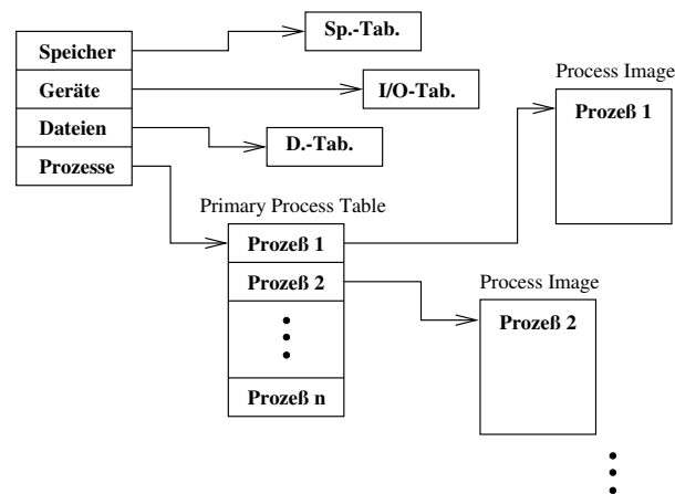
Abbildung 3.15: Struktur der Prozesstabelle
