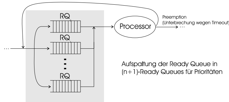
Abbildung 5.1: Aufspaltung in mehrere Ready-Queues für Prioritäten
