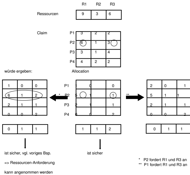
Abbildung 6.9: Beispiel eines unsicheren Zustandes
