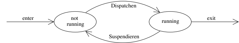
Abbildung 3.7: 2-Zustands-Prozessmodell
