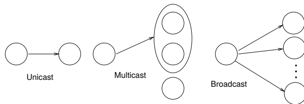
Abbildung 10.1: Grundlegende Verbindungstypen
