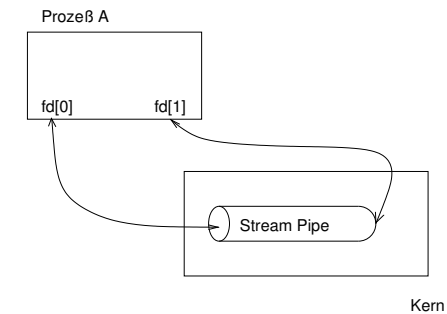
Abbildung 10.11: Stream-Pipe
