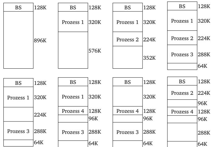
Abbildung 8.3: Dynamische Partitionierung
