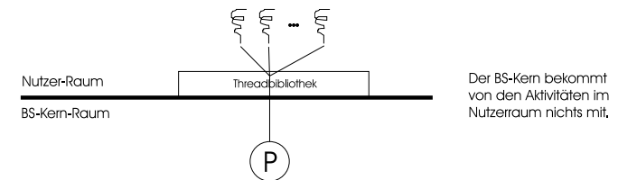
Abbildung 4.5: User-level-Thread-Modell 2
