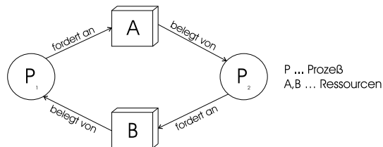
Abbildung 6.7: Circular Wait
