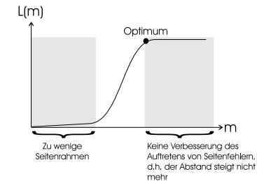
Abbildung 8.12: Lifetime-Funktion L(m)
