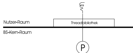
Abbildung 4.4: User-level-Thread-Modell
