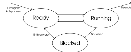
Abbildung 4.3: Thread-Zustandsübergangsdiagramm
