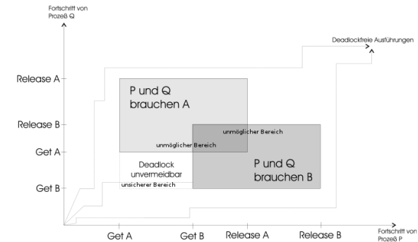
Abbildung 6.4: Prozeßfortschrittsdiagramm 1
