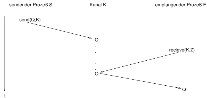
Abbildung 10.2: Send-Receive-Kommunikation (asynchron)
