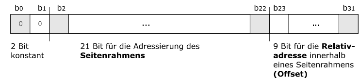
Abbildung 8.9: MI-Maschinenadresse
