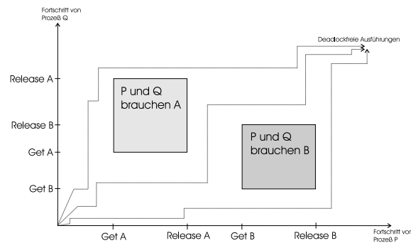
Abbildung 6.5: Prozeßfortschrittsdiagramm 2
