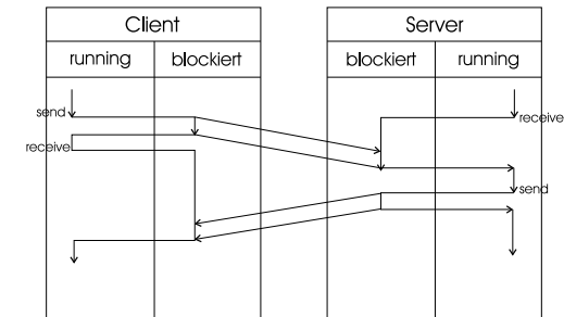
Abbildung 11.9: Blockierende Kommunikationsprimitive
