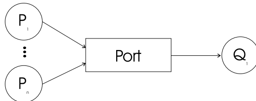
Abbildung 7.11: Indirekte Adressierung n:1
