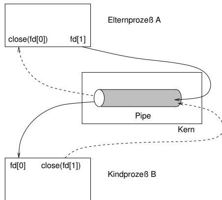
Abbildung 10.7: Daten fließen zum Kindprozeß
