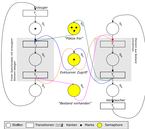
Abbildung 6.17: Petri-Netz zur Modellierung des Erzeuger/Verbraucher-Problems
