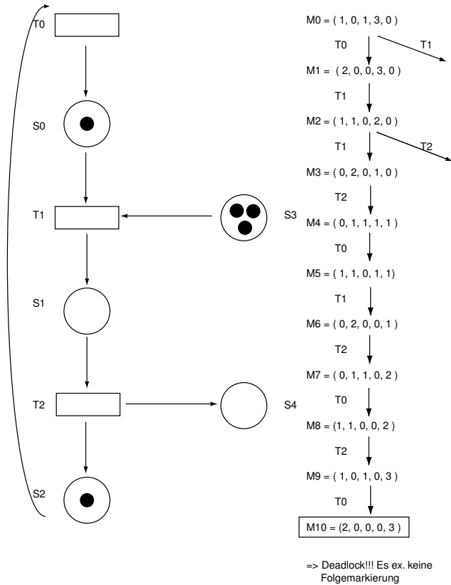
Abbildung 6.23: Beispiel eines Deadlocks
