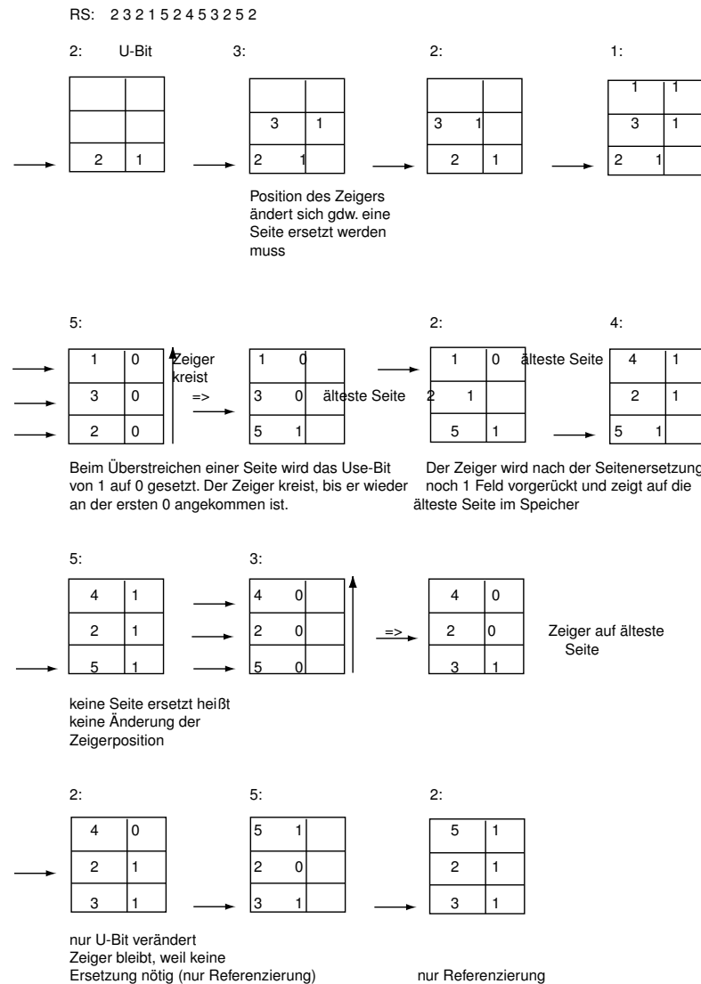
Abbildung 8.11: Beispiel zur Clock-Strategie
