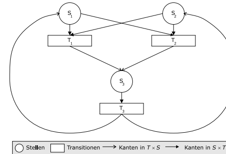
Abbildung 6.10: Beispiel für ein Petri-Netz
