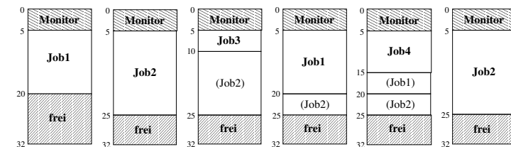
Abbildung 3.16: Beispiel: Speicherbelegung bei CTSS
