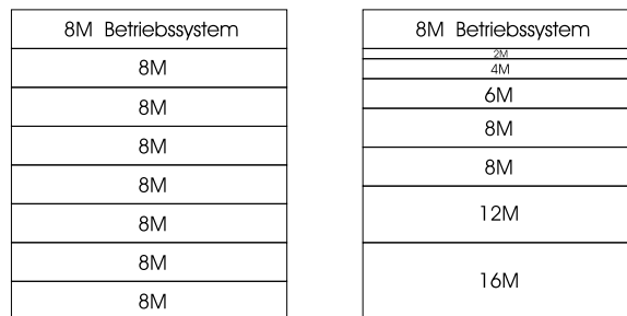
Abbildung 8.1: Beispiel für feste Partitionierung
