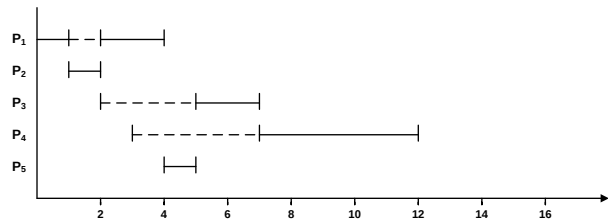
Abbildung 5.5: Beispiel mittlere Verweildauer für SRPT
