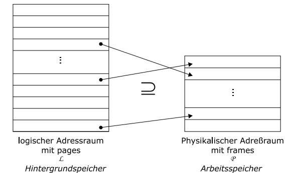
Abbildung 8.8: Abbildung zwischen frames und pages
