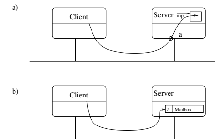
Abbildung 11.11: ungepufferte und gepufferte Primitive
