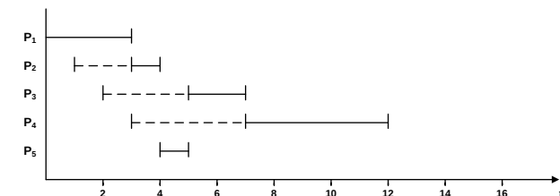
Abbildung 5.3: Beispiel mittlere Verweildauer für SJF
