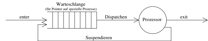
Abbildung 3.8: Warteschlangenmodell des 2-Zustand-Prozessmodells
