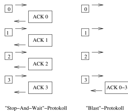
Abbildung 11.16: Möglichkeiten zur Bestätigung
