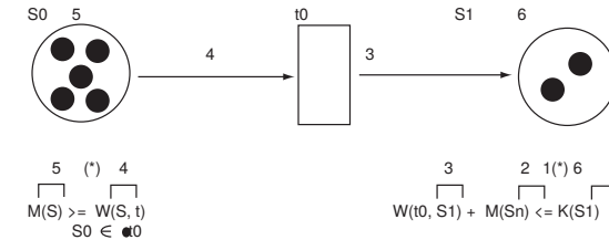
Abbildung 6.14: Stellen-Transitionssystem mit Markierungen
