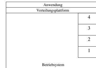
Abbildung 11.3: Einordnung der Verteilungsplattform in die Softwarearchitektur
