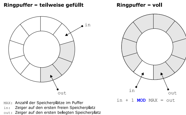
Abbildung 7.2: Darstellung eines einfachen Ringpuffers
