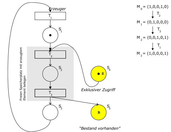
Abbildung 6.26: Entstehen eines Deadlocks
