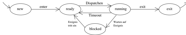
Abbildung 3.9: 5-Zustands-Prozessmodell
