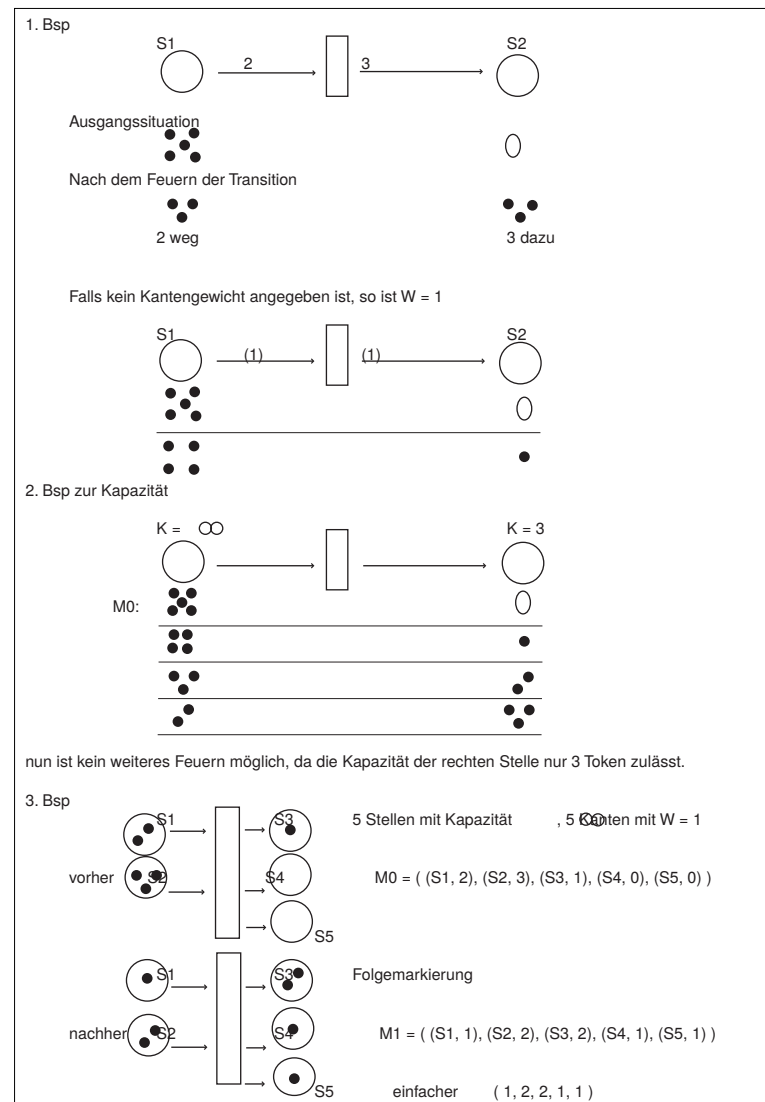
Abbildung 6.11: Stellen-Transitionssysteme
