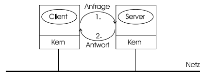
Abbildung 11.4: Das Client/Server-Modell
