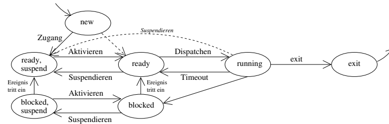
Abbildung 3.13: 7-Zustands-Prozessmodell
