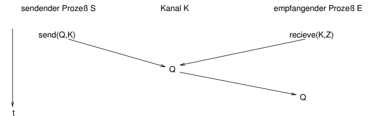
Abbildung 10.4: Synchrone Kommunikation
