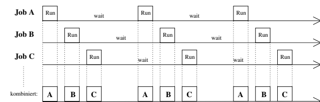
Abbildung 3.2: Pseudo-parallele Ausführung
