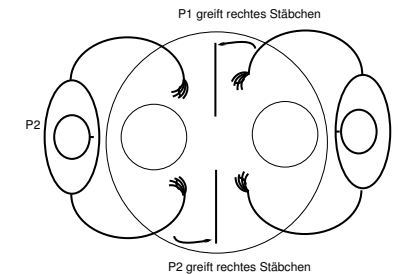
Abbildung 6.2: Beispiel Philosophenproblem
