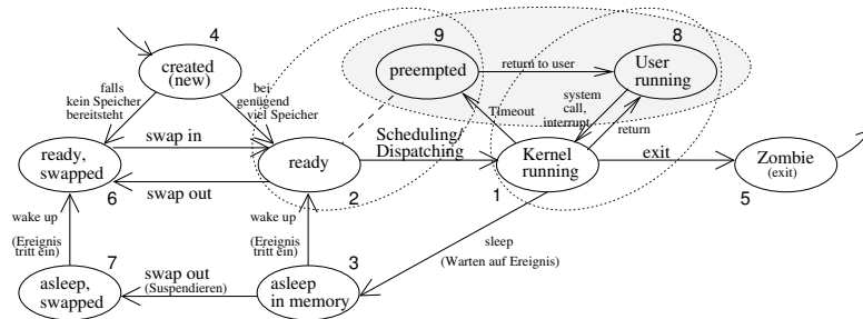
Abbildung 3.29: 9-Zustands-Modell (UNIX)
