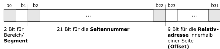
Abbildung 8.10: MI-Programmadresse
