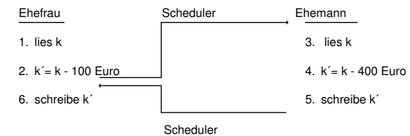
Abbildung 5.4: Programmbefehle
