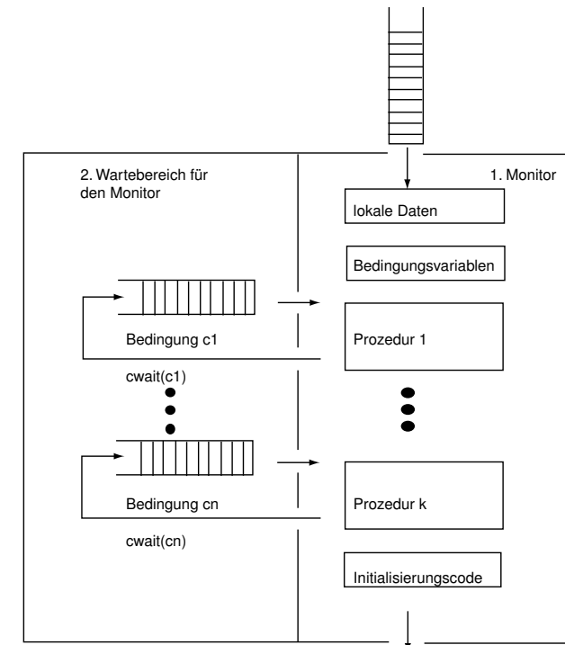
Abbildung 7.8: Monitor
