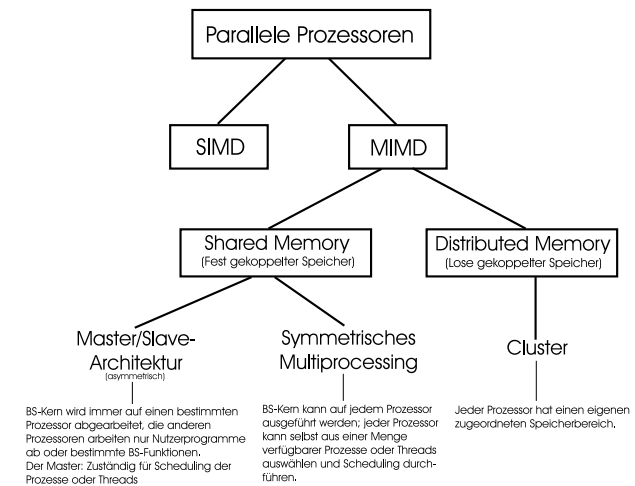
Abbildung 4.9: Parallele Prozessoren
