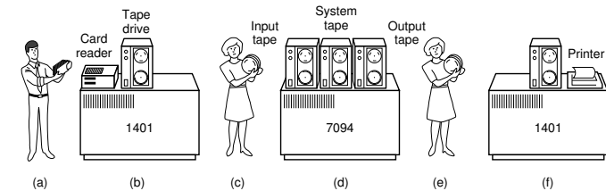
Abbildung 1.2: Erste Stapelverarbeitungssysteme
