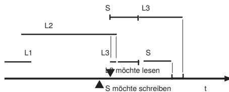
Abbildung 6.18: R/W-Problem
