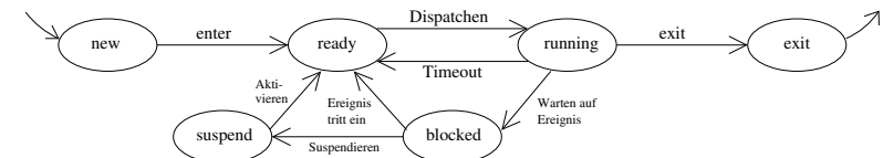
Abbildung 3.12: 5-Zustands-Modell mit Suspend
