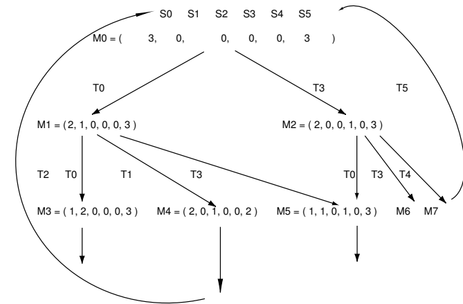
Abbildung 6.21: Erreichbarkeitsgraph zum R/W-Problem
