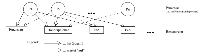
Abbildung 3.14: Verwaltung der Nutzung von Systemressourcen
